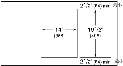
工作台面开孔尺寸
