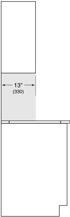
侧视图
