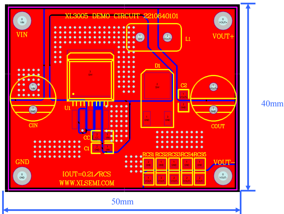
顶层
