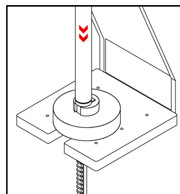
9. Bajar pistón
