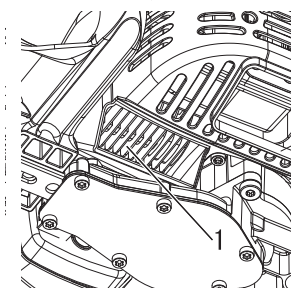
1. Aletas del cilindro
