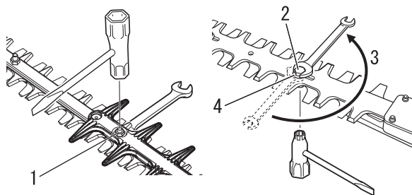
1. Gegenmutter 2. Schraube
