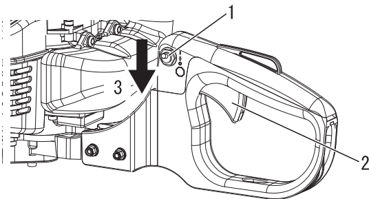
1. Zündschalter 2. Gashebel
