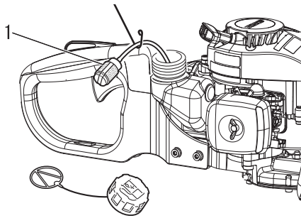
1. Kraftstofffilter
