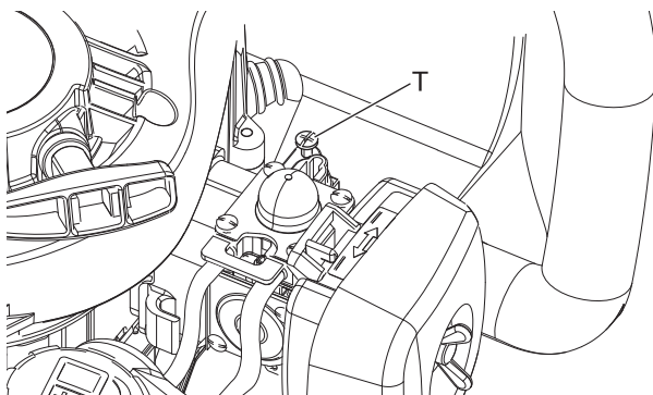
T: Regulador de velocidad de ralentí
