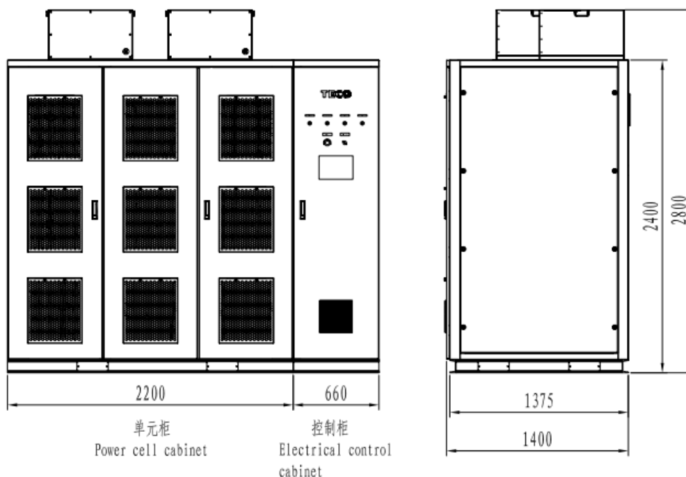
图 3-1 控制柜和单元柜外形图
