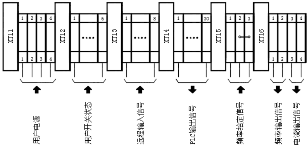
图 3-18 变频器与用户的信号接口图
