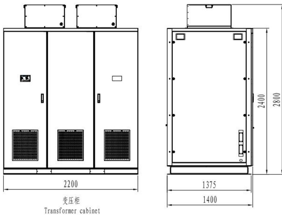
图 3-3 变压器柜外形图
