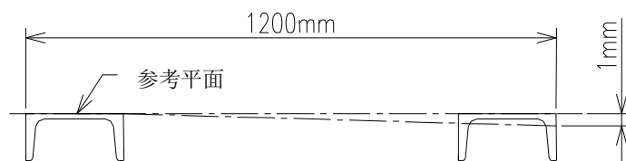
图 3-8 垂直容差图
