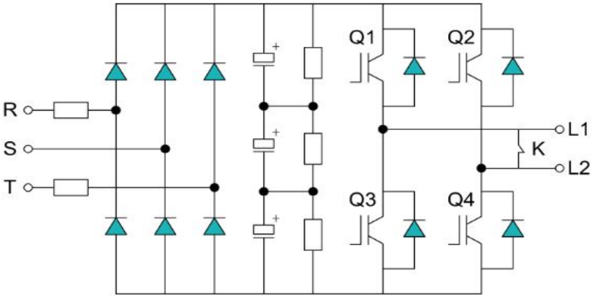
图 5-3 功率单元结构图
