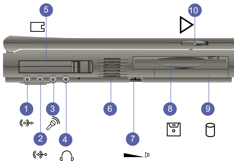
圖1-5 左視圖
