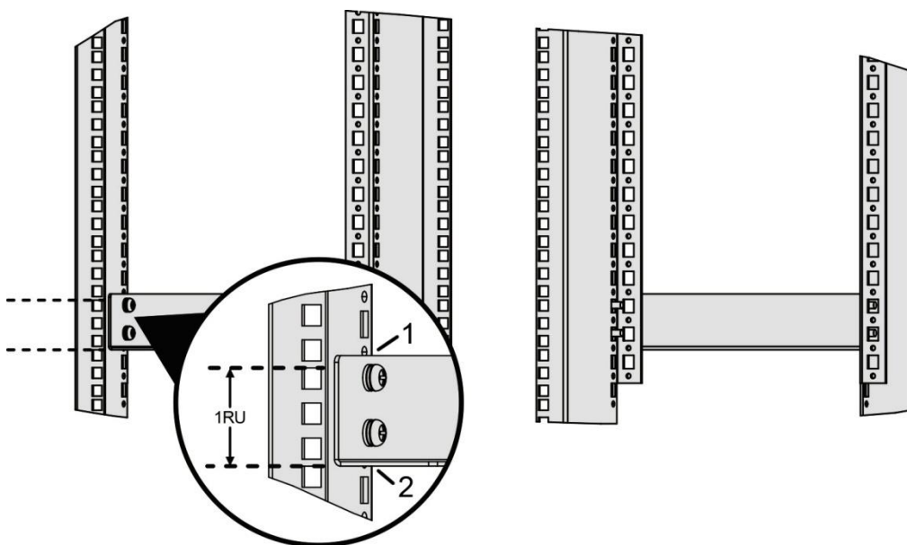
图 4-3 滑道示意图
