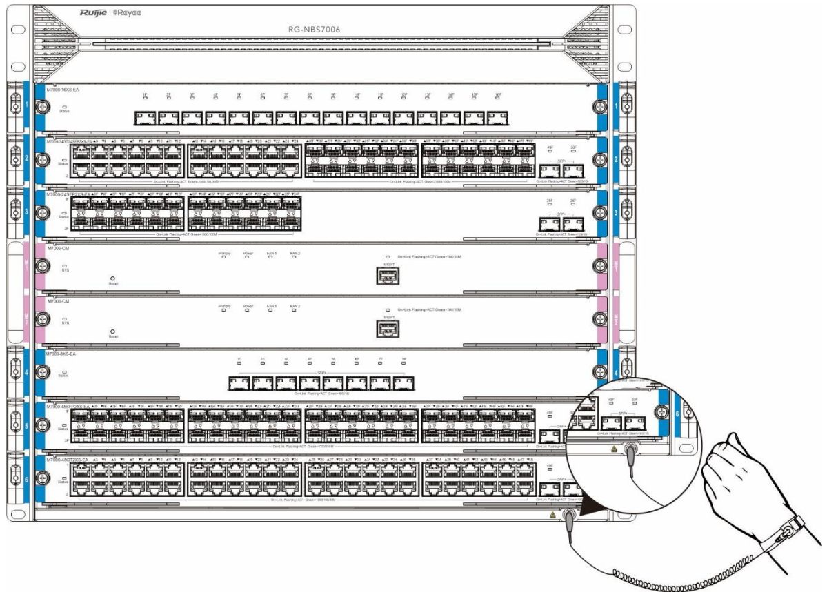
图 3-2 RG-NBS7006 防静电方式示意图
