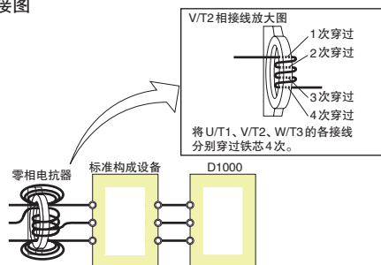
连接图a
