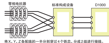
连接图c
