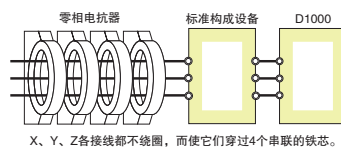
连接图b
