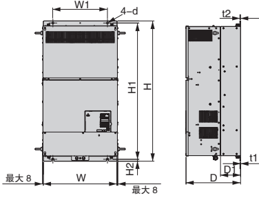
外形图2
