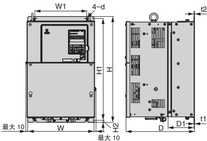
外形图1
