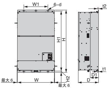
外形图3
