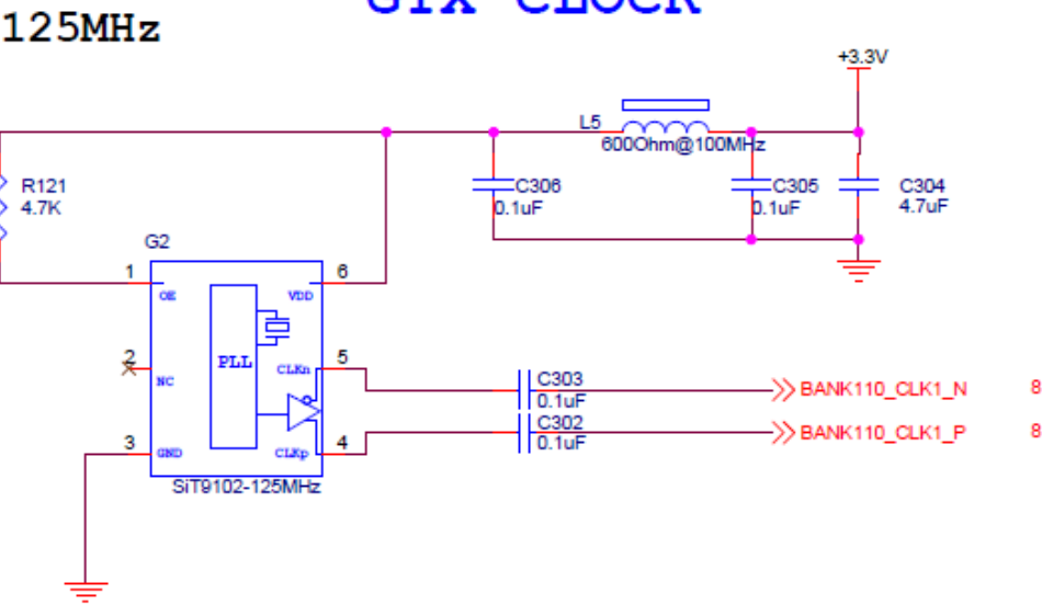
图 2-6-6 GTX 时钟源
