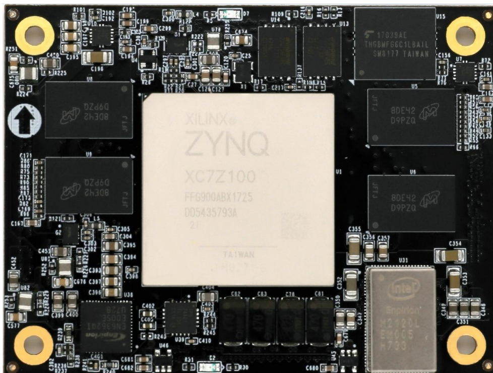
AC7Z100 核心板正面图
