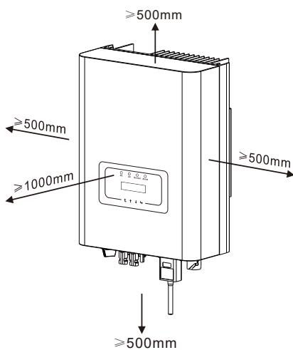
Figura 4.3 Espaçamento de Instalação
