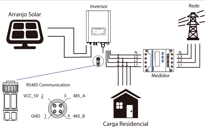
Figura 7.12 Conexão do diagrama do medidor CHINT
