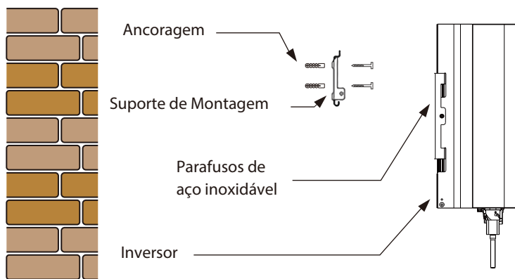
Figura 4.4 Instalação do Inversor
