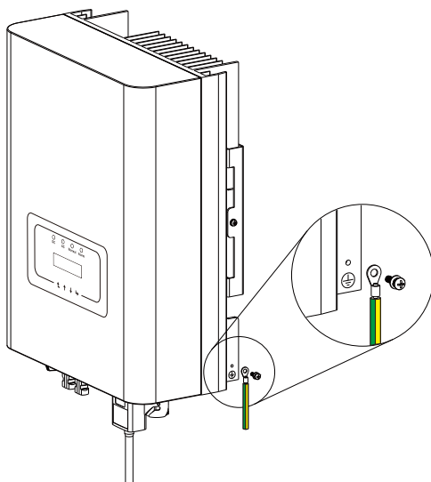
Figura 5.11 A instalação do Aterramento da Carcaça
