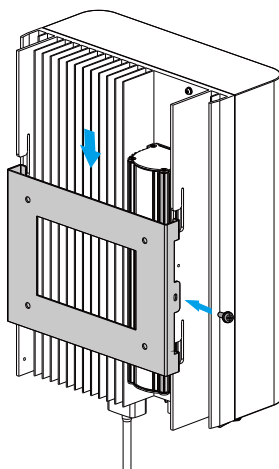
Figura 4.6 Instalação do Inversor
