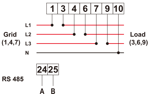
Figura 7.11 Medidor CHINT
