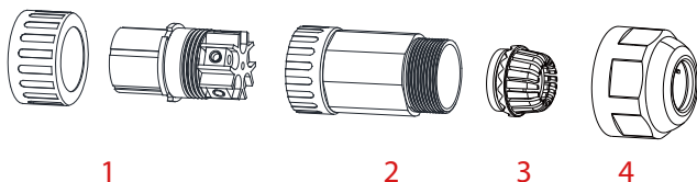
1. Soquete de Encaixe 2. Luva 3. Núcleo de Selamento 4. Porca de Selamento
