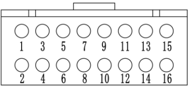
图 2-2 输入输出管脚（母座）
