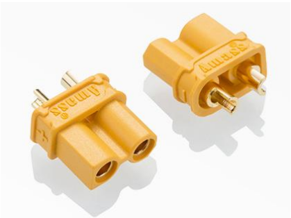
图 2-1 UM 一体伺服的供电端子
