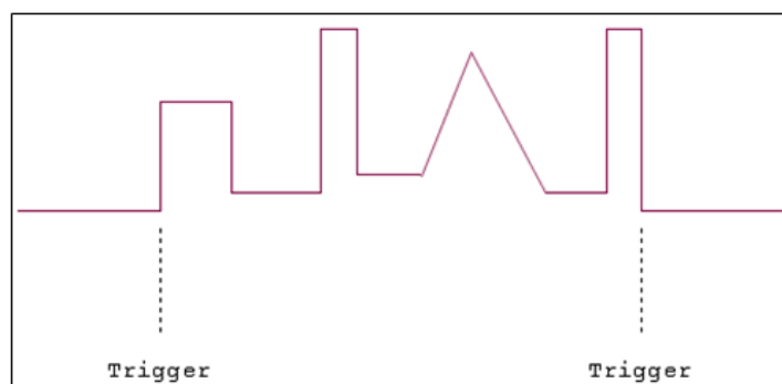
LIST 输出波形示意图
