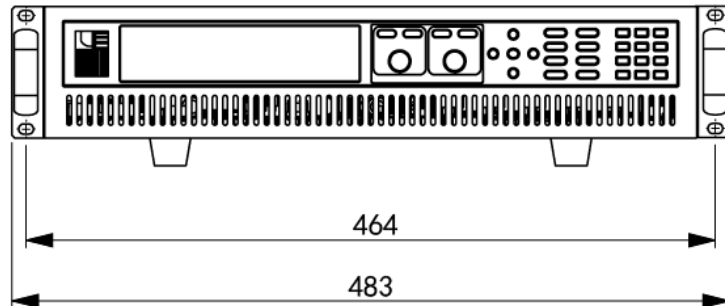
详细尺寸图
