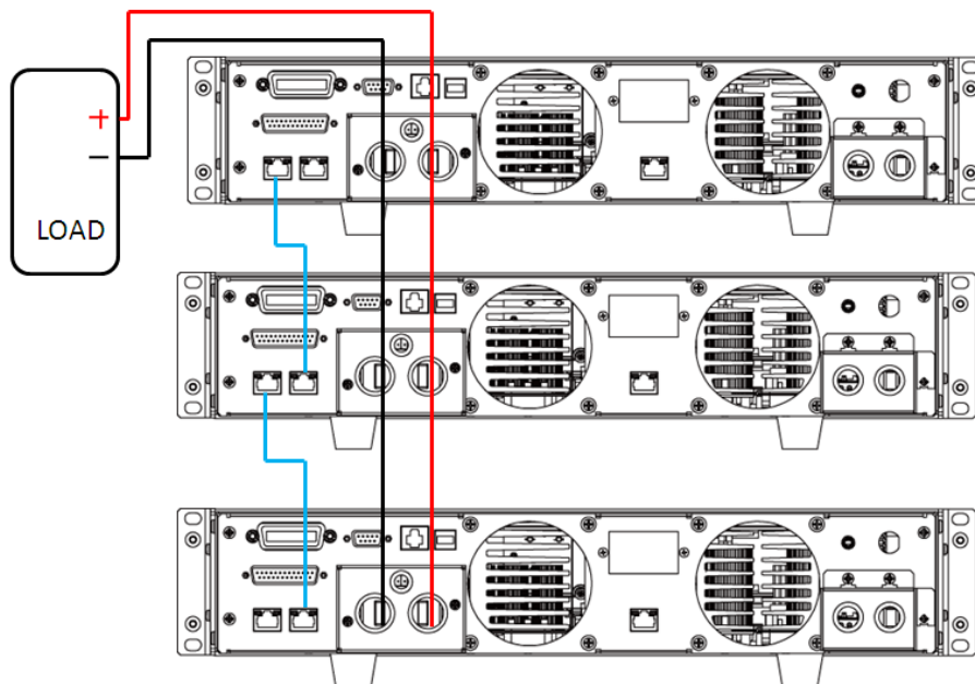
图 1 三台并联的电源设备示意图
