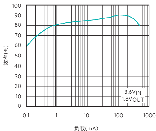
高效率(MAX8640Y)
