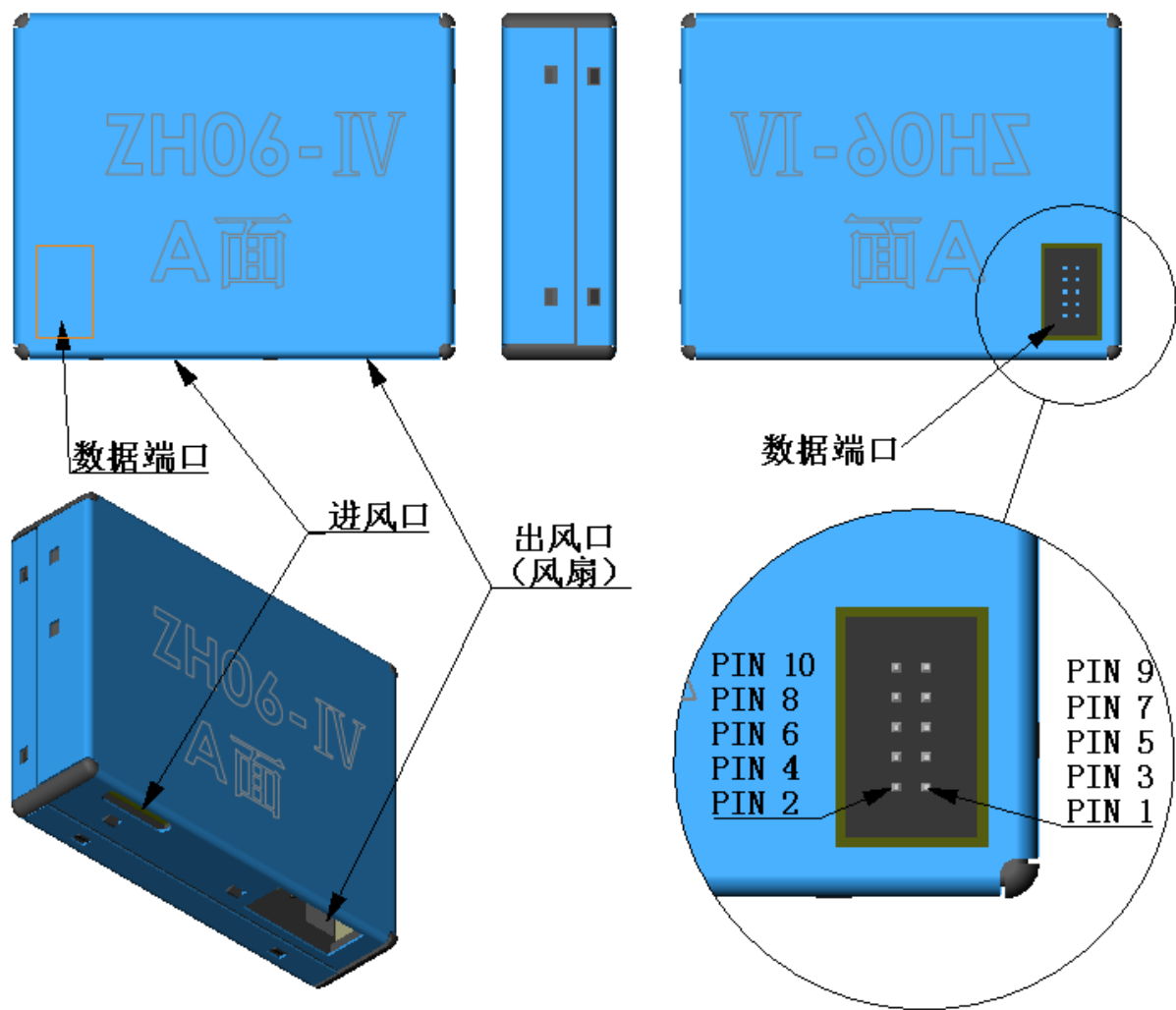
图 1-引脚顺序
