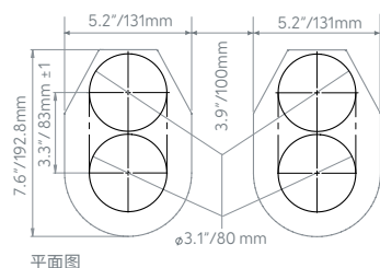
平面图
