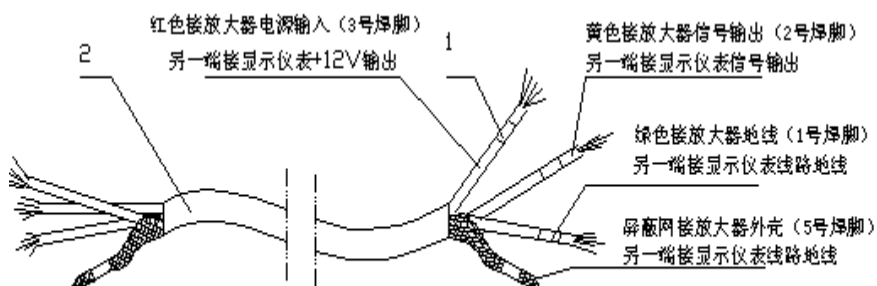
图三 LWGY—50~200 传感器结构及安装尺寸示意图
