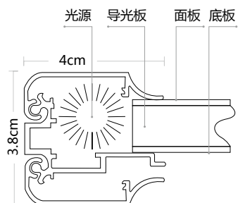
侧面双开图
