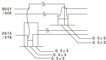
并行接口信号时序图
