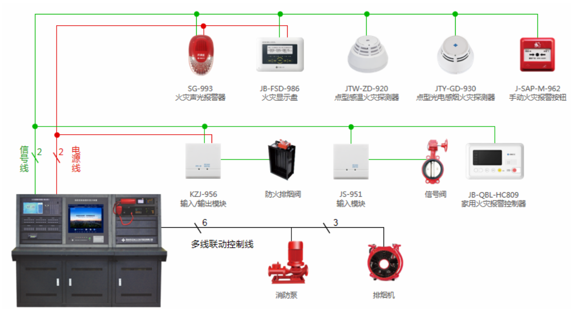
三江电子火灾自动报警及消防联动控制系统主要组件如下：
