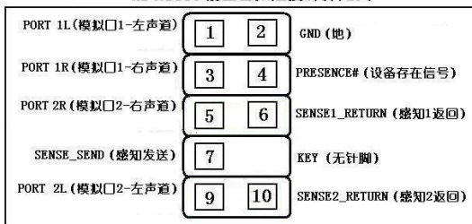
AC97 与 HD 音频连接座针脚定义对比表
