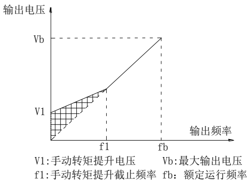
图 5-11: 手动转矩提升示意图
