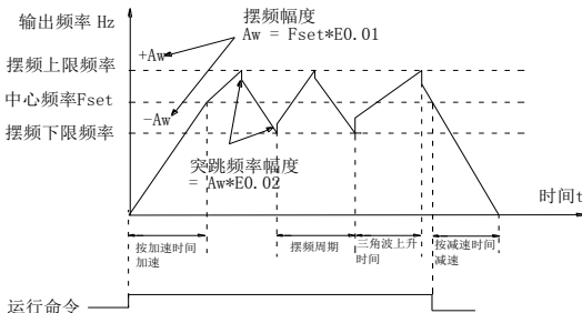
图 5-28: 摆频工作示意图
