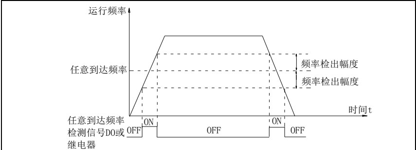
图 5-23：任意到达频率检测示意图
