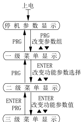
图 3-2: 操作流程图
