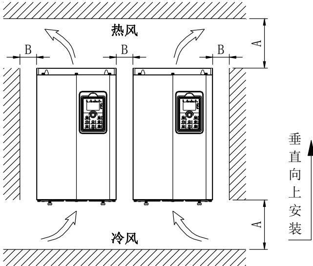
图4-1:PI510 系列各功率等级安装空间要求
