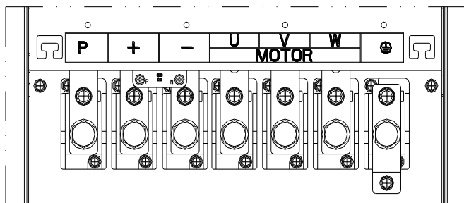
图4-4:45kW~75kW G3 主回路端子图
