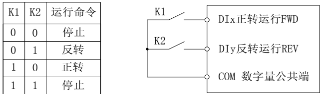
图 5-3：端子命令方式：两线制模式 1
