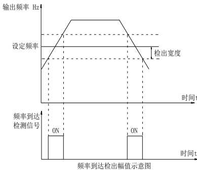
图 5-22: 频率到达检出幅值示意图
