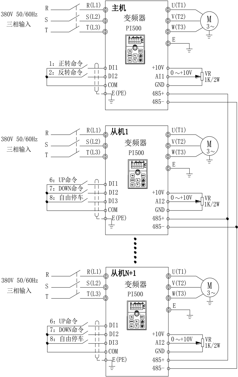
图 II-1：系统接线图
