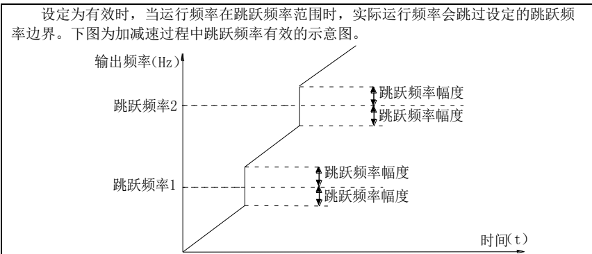
图 5-18: 加减速过程中跳跃频率有效示意图
