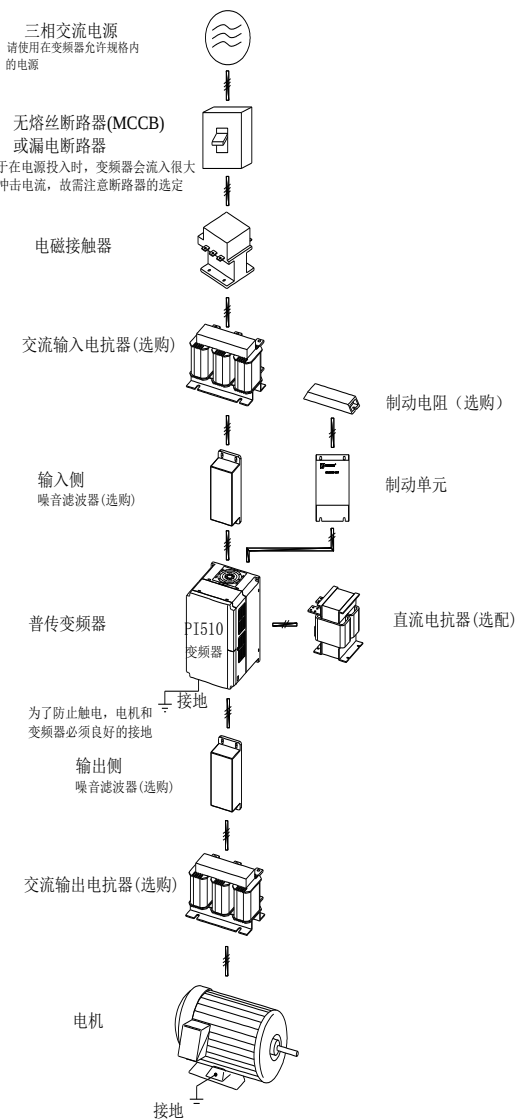
图 9-1：选件接线图
