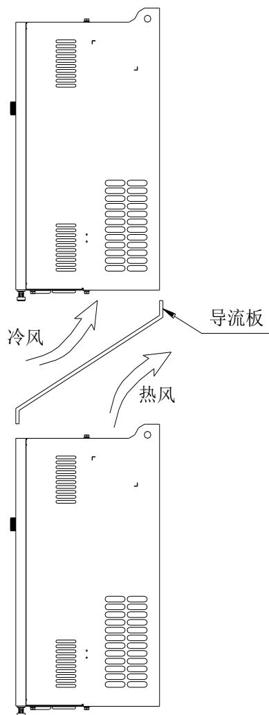
图4-2:隔热导流板安装示意图上下安装图
