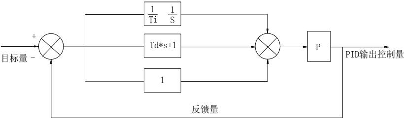
图 5-31：过程 PID 原理框图
