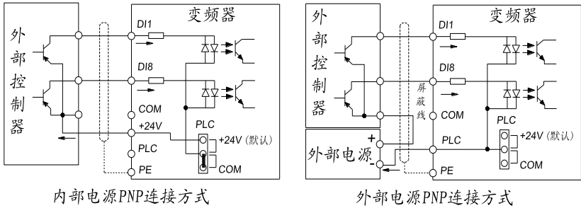
图4-12：信号输入端子接线图—开路集电极 PNP 接线方式
