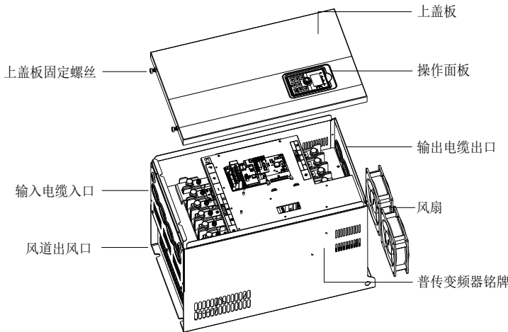
图7-1：产品外型图、安装孔位尺寸
