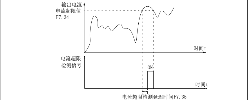
图 5-25：输出电流超限检测示意图
