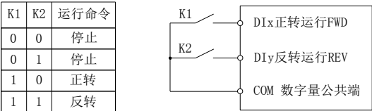
图 5-4：端子命令方式：两线制模式 2
