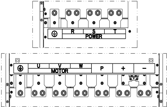
图4-8:250kW~400kW G3 主回路端子
