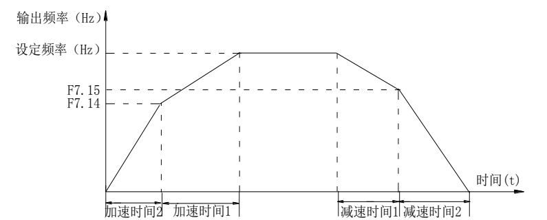
图 5-19: 加减速时间切换示意图
