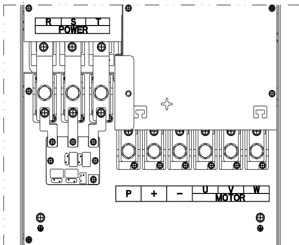
图4-5:93kW~110kW G3 主回路端子图
