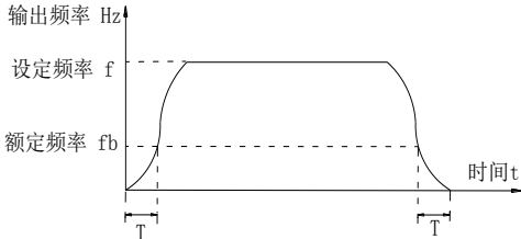
图 5-10: S 曲线加减速 B 示意图
