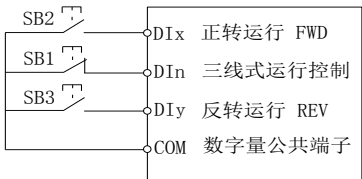
图 5-5：端子命令方式：三线制控制模式 1
