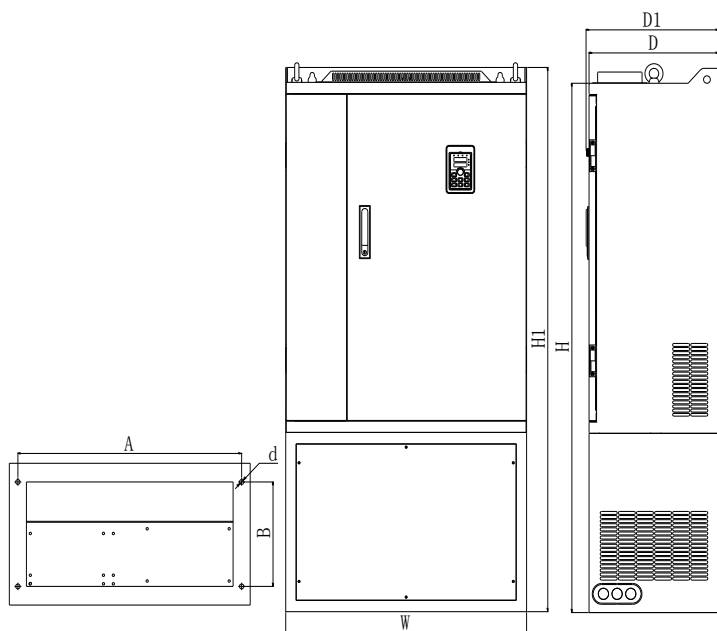
图7-6: 250kW~400kW(带有直流电抗器底座)外形尺寸
