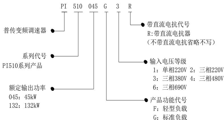
图 1-2：型号说明
