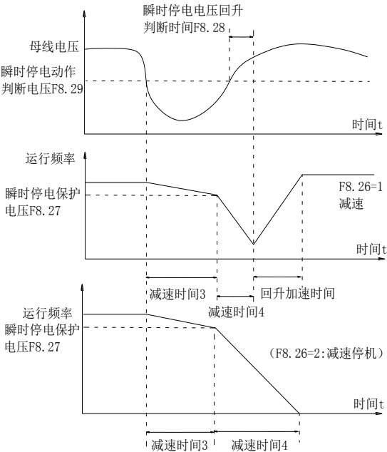
图 5-27：瞬时停电动作示意图
