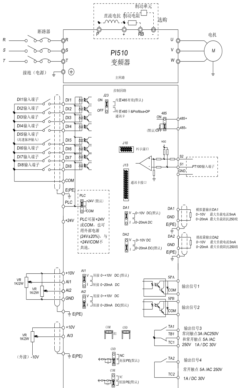
图4-3: 配线图
