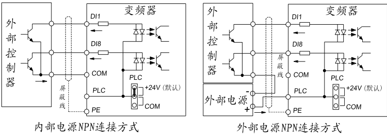
图4-11: 信号输入端子接线图—开路集电极 NPN 接线方式
