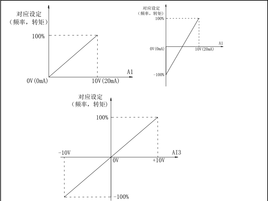
图 5-7：模拟给定与设定量的对应关系
