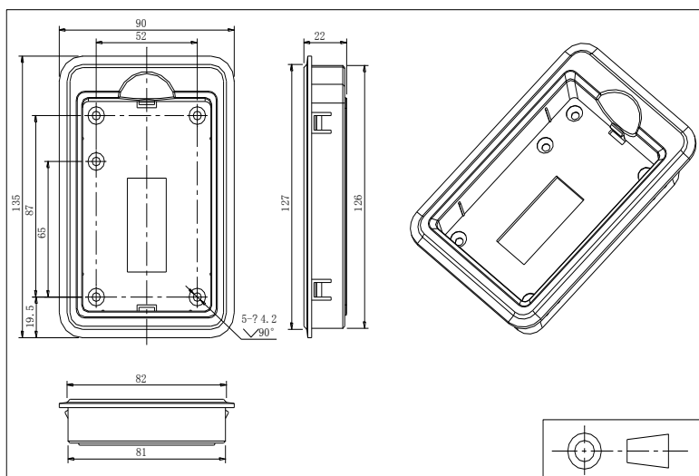
图7-8: 键盘仓尺寸图 (尺寸单位: mm)
