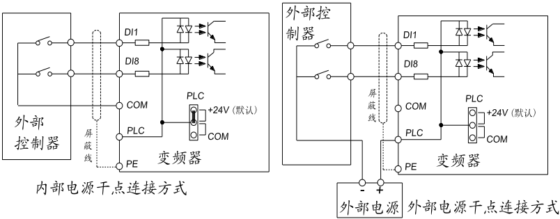
图4-10: 信号输入端子接线图—干接点方式
