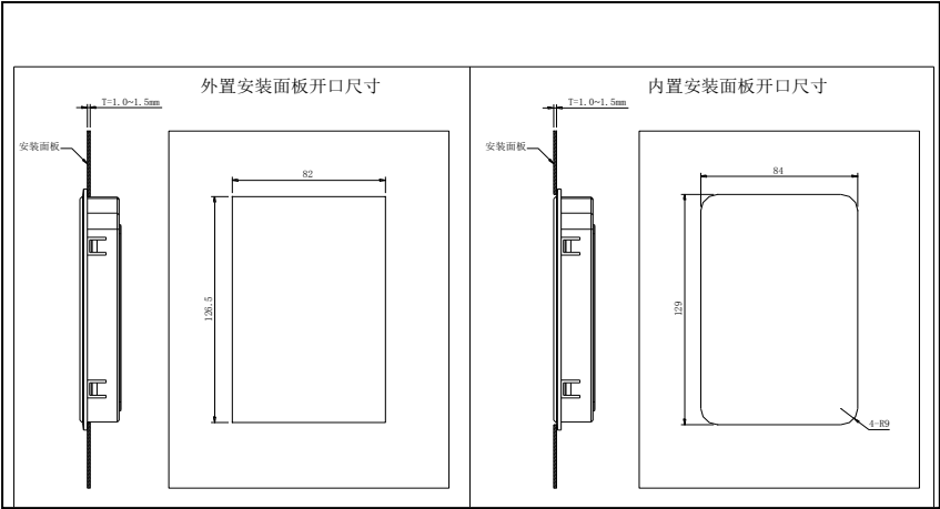
图7-9: 键盘安装开口尺寸图(尺寸单位: mm)
