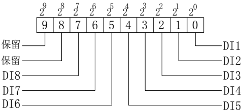
图 5-1：DI 输入状态端子顺序
