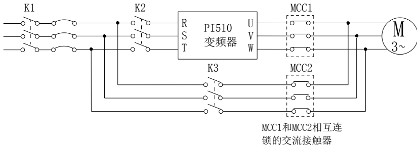
图4-13: 备用电路电气图
