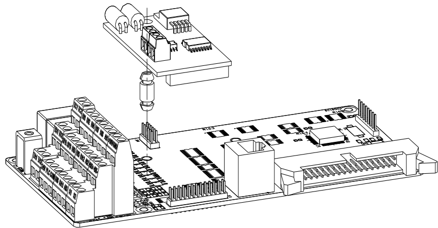
图 IV-1：CAN 总线通信卡在 PI510 控制板上的安装
