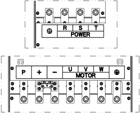
图4-6:132kW G3 主回路端子
