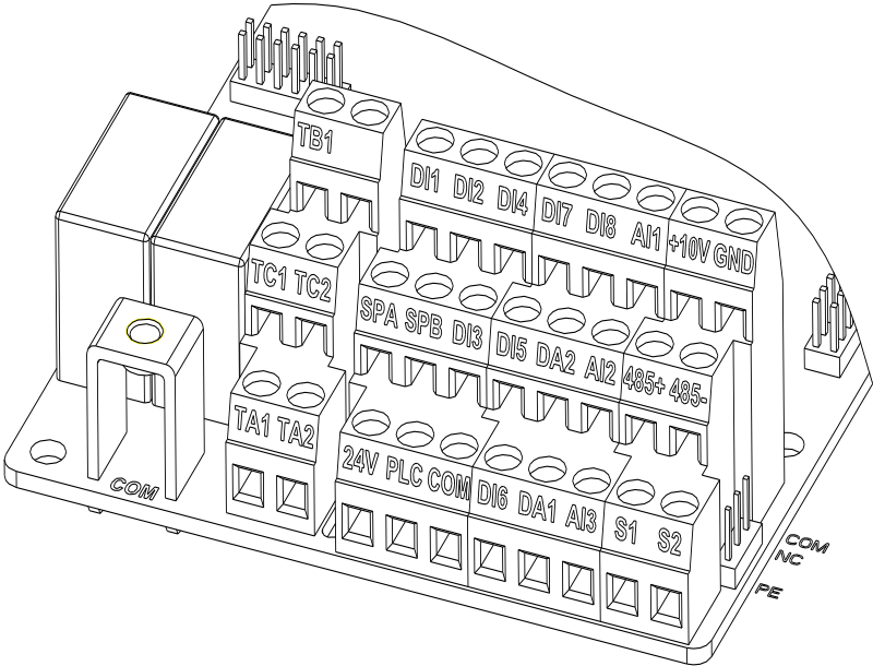
图4-9:控制板控制回路端子
