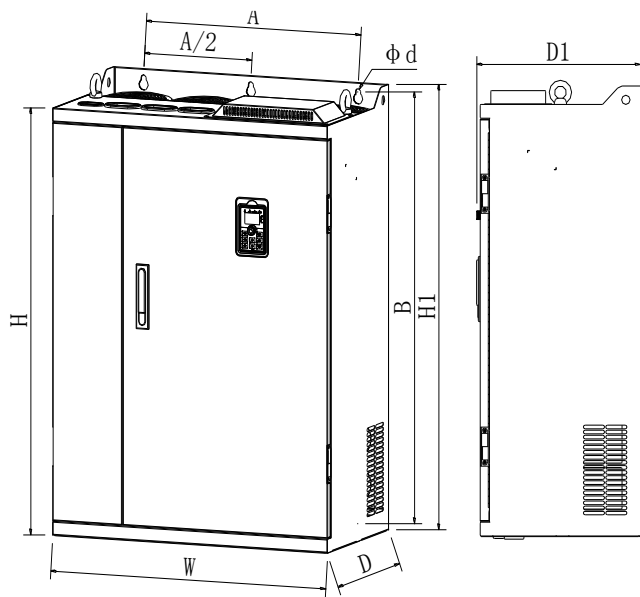
图7-3：250kW~400kW 外形尺寸
