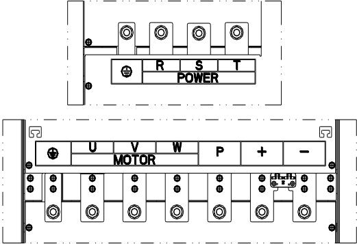
图4-7:160kW~220kW G3 主回路端子
