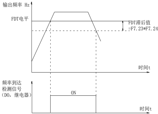
图 5-21: FDT 电平示意图
