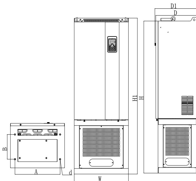
图7-5: 160kW~220kW(带有直流电抗器底座)外形尺寸
