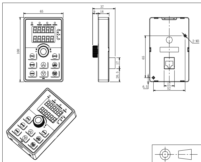
图7-7: PI510 键盘尺寸图 (尺寸单位: mm)
