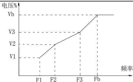
V1-V3:多段速V/F第1-3段电压百分比 F1-F3:多段速V/F第1-3频率 Vb:电机额定电压 Fb:电机额定运行频率
