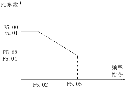
图 5-13：PI 参数示意图
