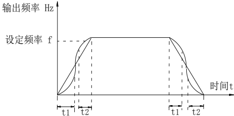
图 5-10: S 曲线加减速 A 示意图
