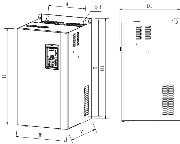
图7-2：45kW~220kW 外形尺寸
