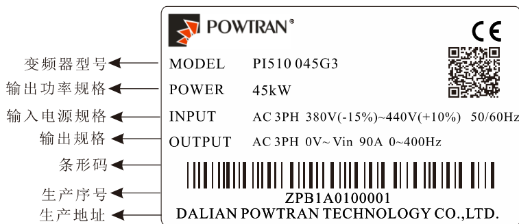
图 1-1：铭牌说明
