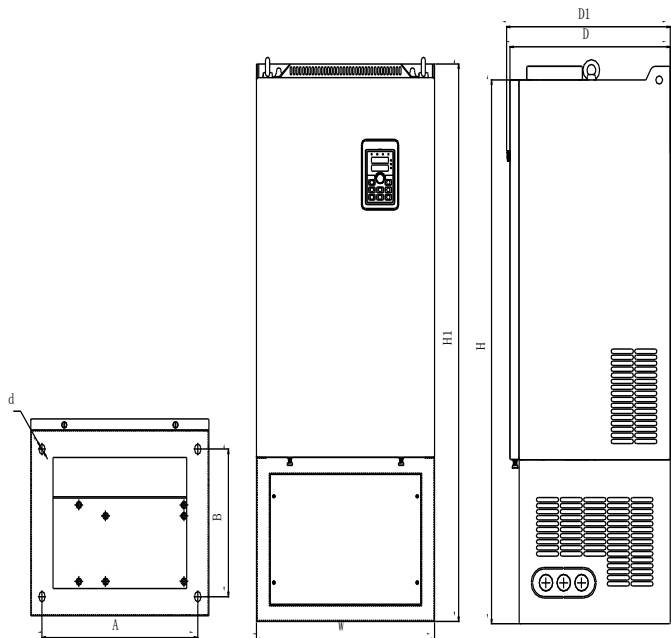
图7-4：132kW(带有直流电抗器底座) 外形尺寸
