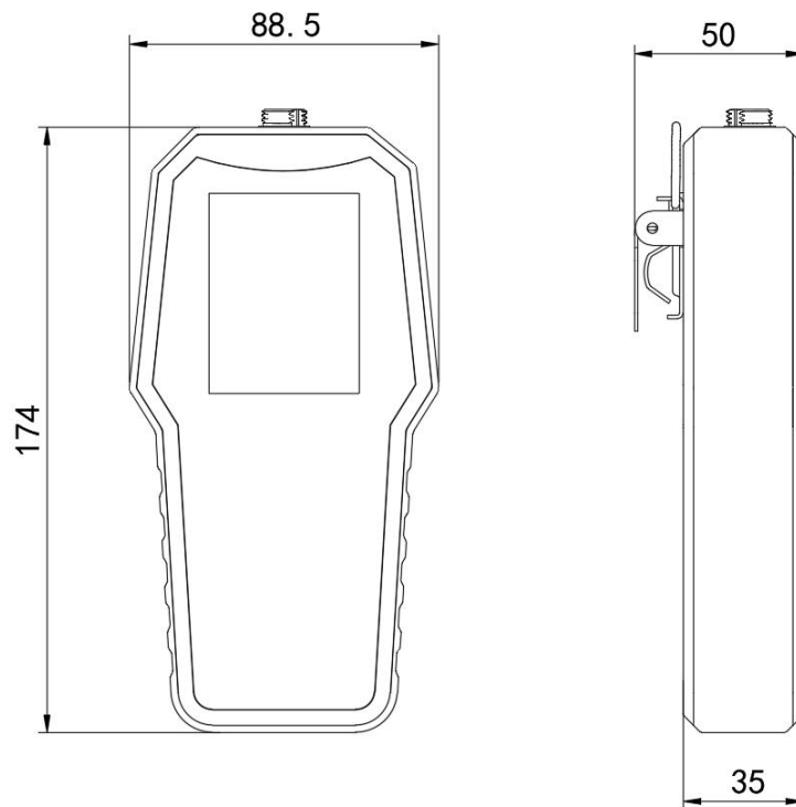
设备尺寸图（单位：mm）
