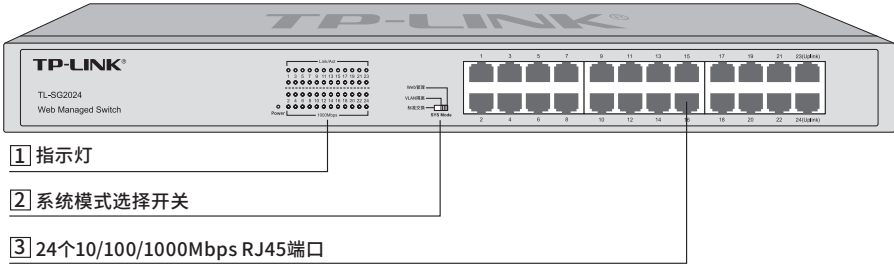
图1-3 TL-SG2024前面板示意图
