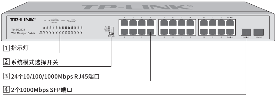
图1-1 TL-SG2226前面板示意图
