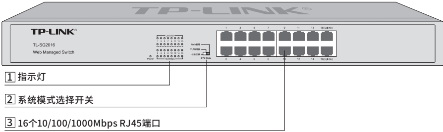
图1-4 TL-SG2016前面板示意图
