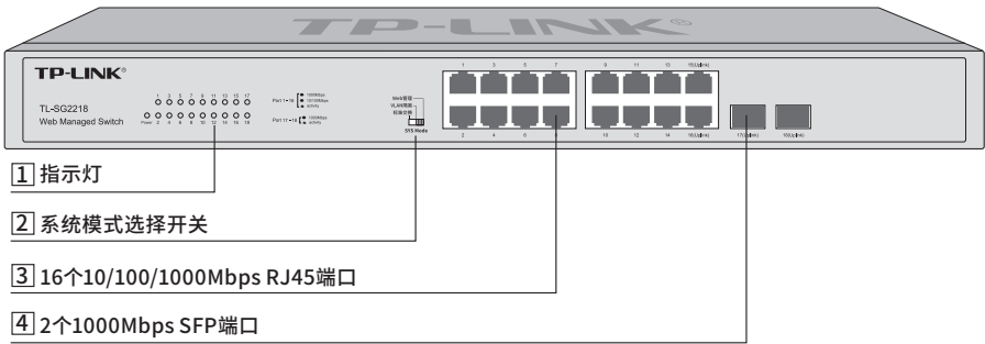
图1-2 TL-SG2218前面板示意图
