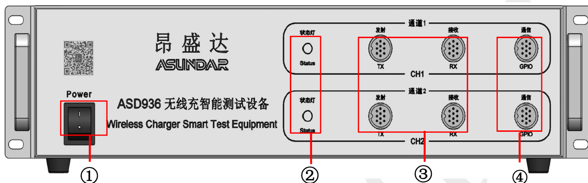
① 电源按钮 ② 状态灯 ③ 测试接口 ④ 通讯接口
