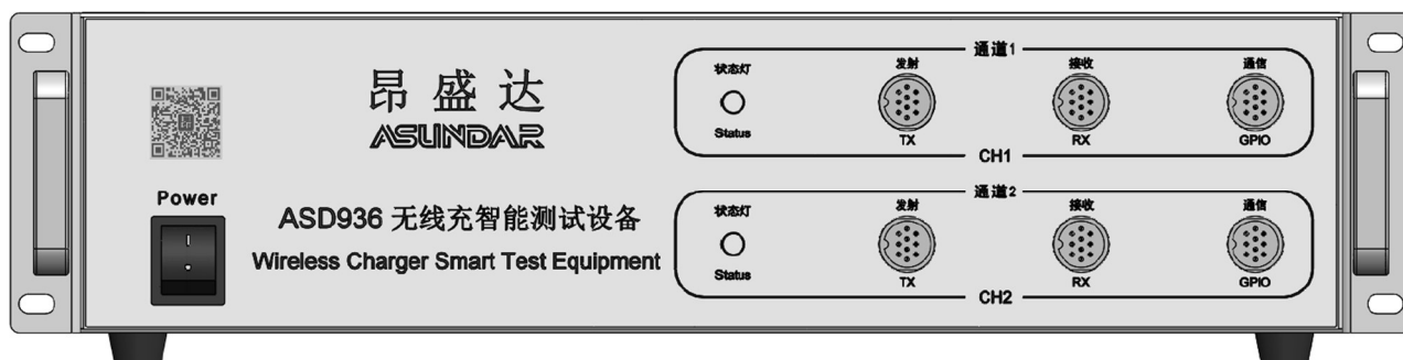
图 2.2: ASD936 前面板
