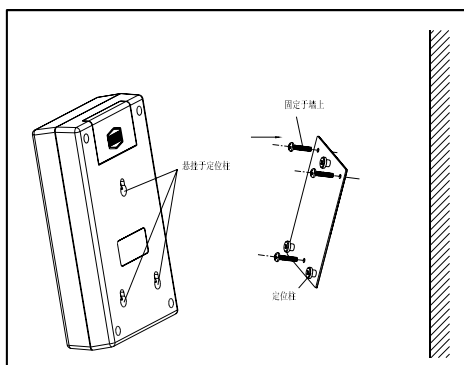
图 3 TPK492C 的安装
