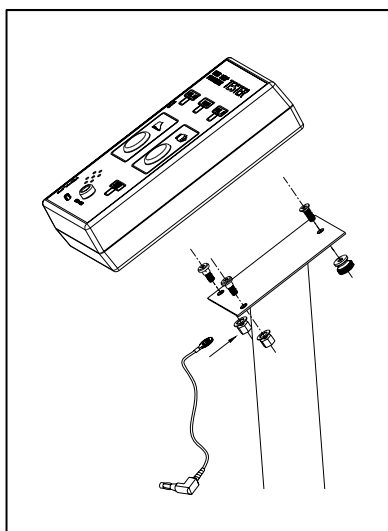
图 2 TPK492B 安装
