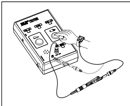
图 5 手腕带的测量
