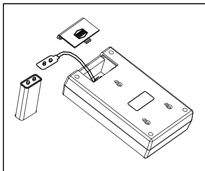
图 4 电池的更换
