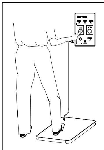
图 6 脚环的测量
