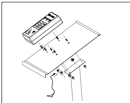
图 1 TPK492A 安装
