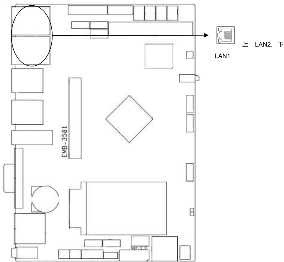
RJ45 LAN LED 状态描述:
