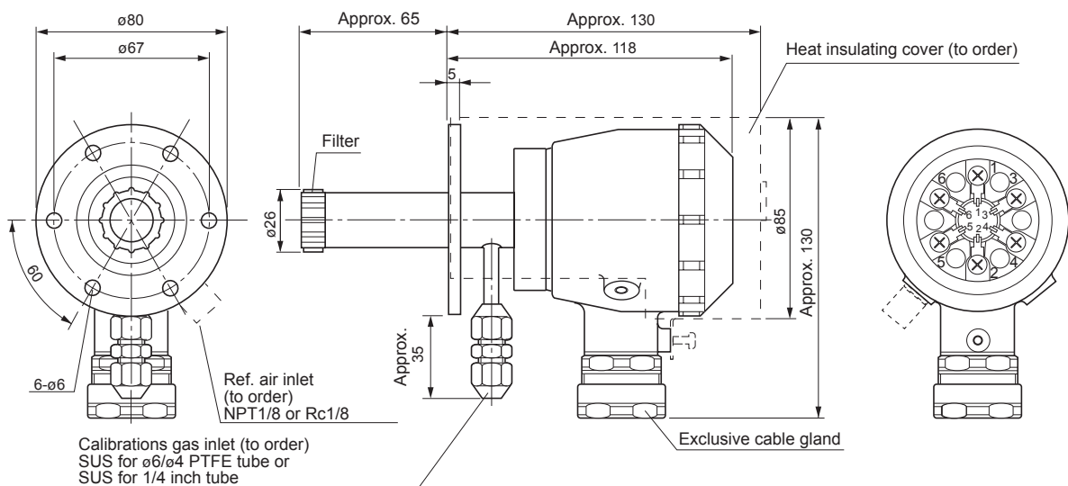
(2) Detector (ZFK5)
