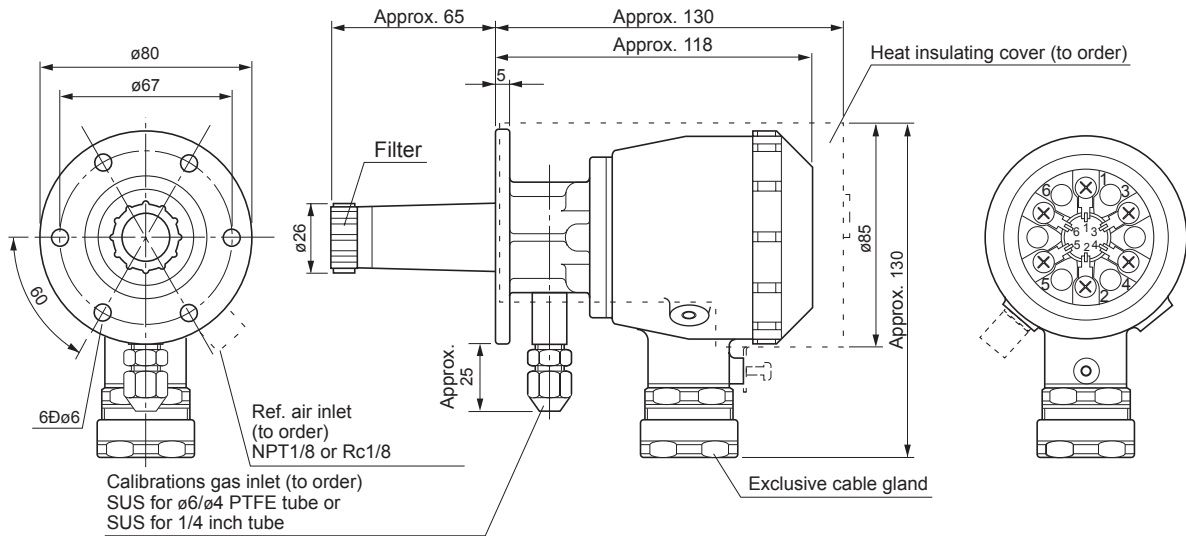
(2) Detector (ZFK5)
