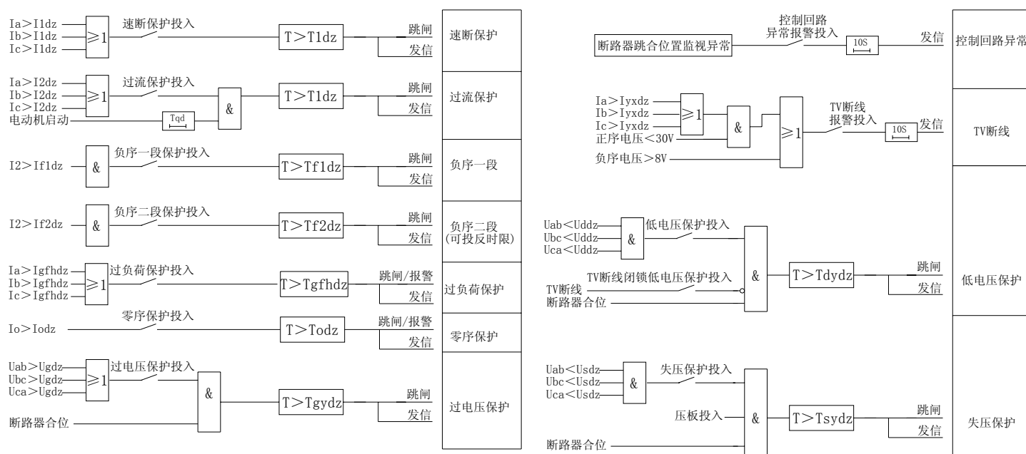
附图5.1 XZ-6141电动机保护测控装置逻辑图
