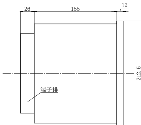
附图二：装置面板布置图
