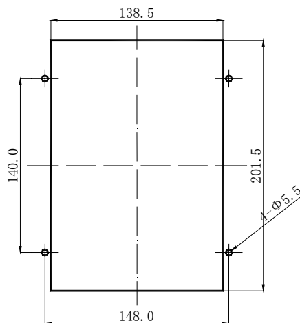
附图四：装置开孔尺寸图
