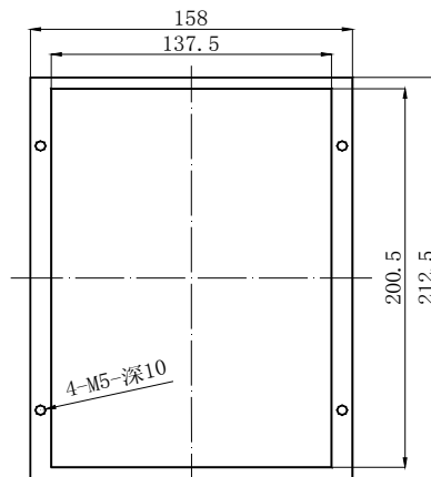
附图四：装置开孔尺寸图
