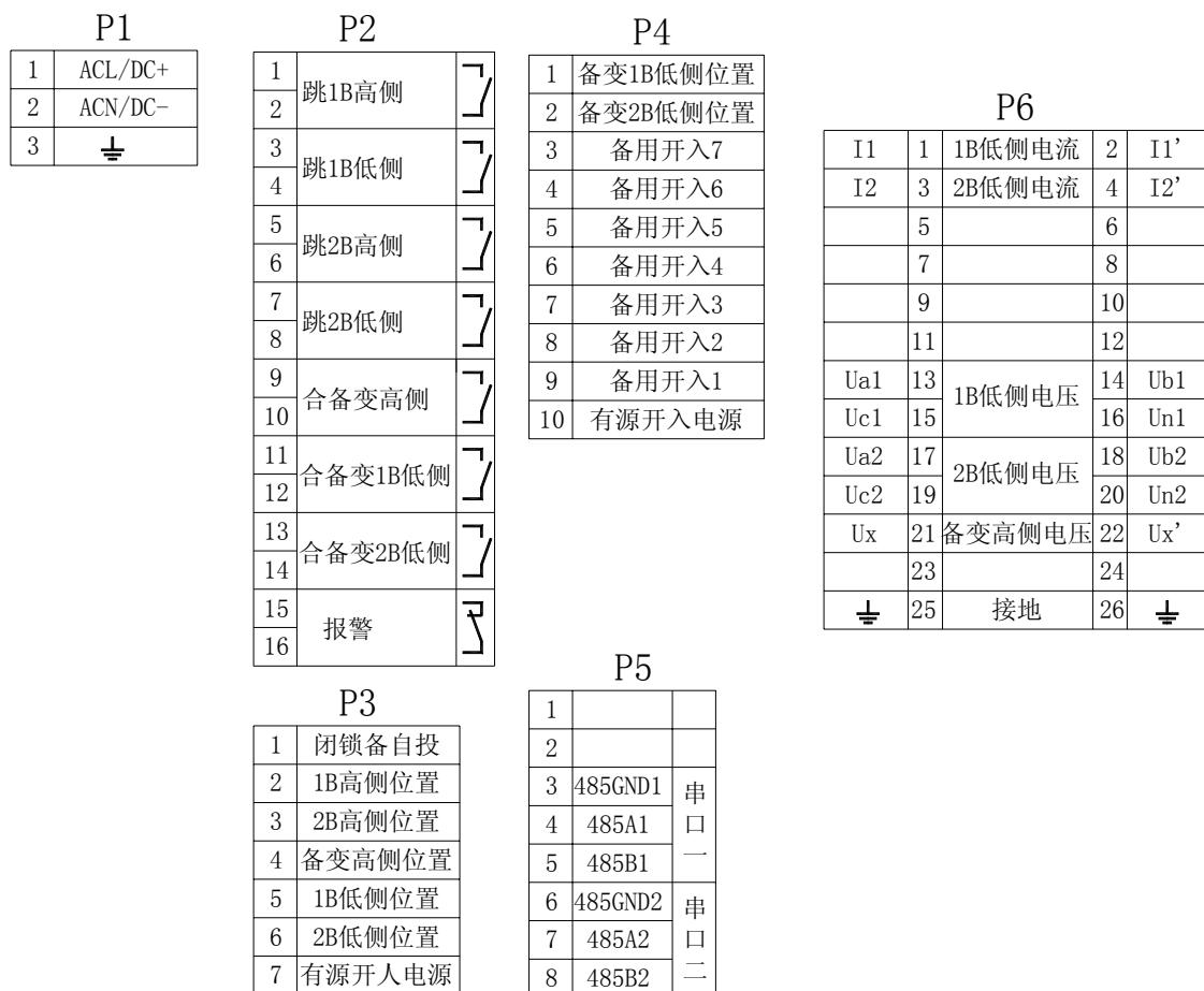
附图8.1 XZ-6162厂用变备自投装置背板端子图
