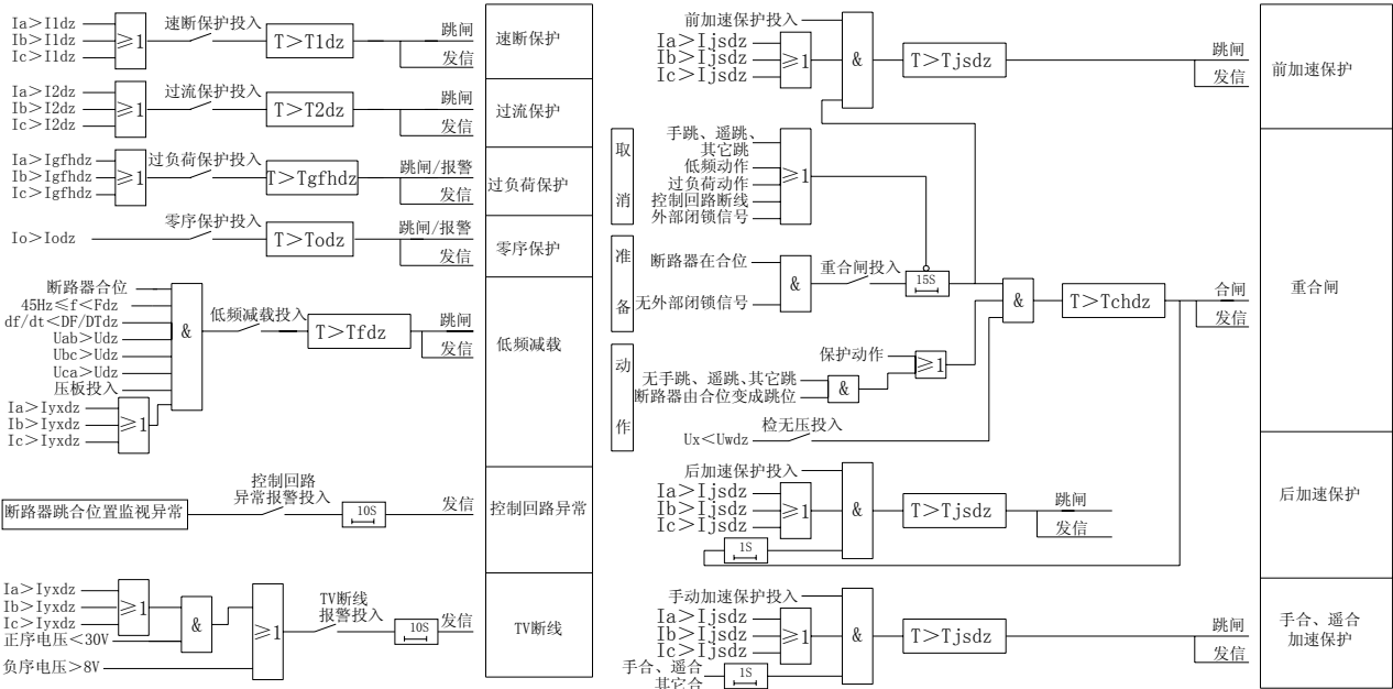
附图2.1 XZ-6111馈线保护测控装置逻辑图
