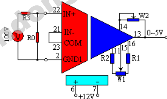
图 4 测量高电压信号
