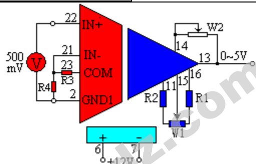
图 3 小信号隔离放大变送
