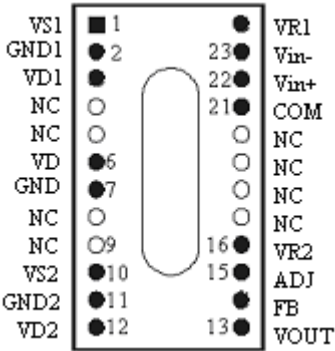
图 6 引脚定义
