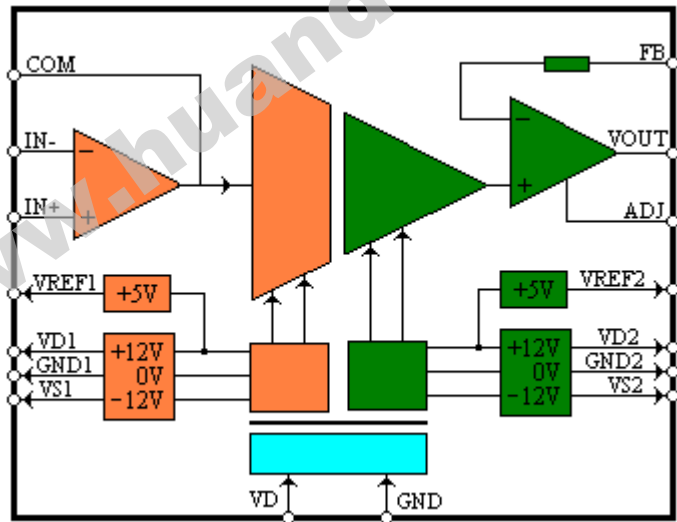
(图 1 原理框图)
