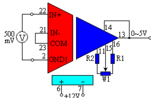
图 2 典型接线图
