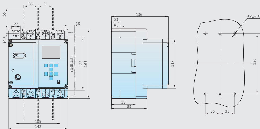
NM2LC-250外形及安装尺寸
