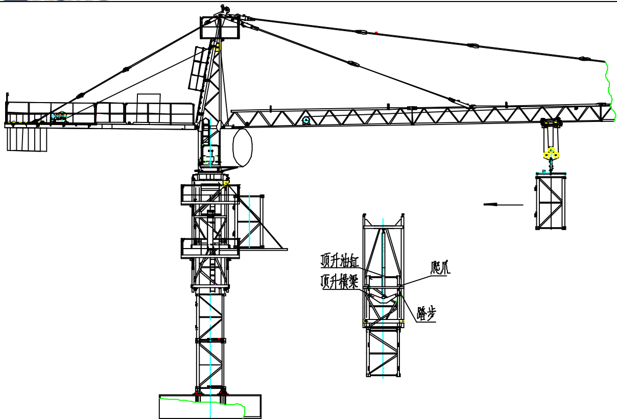
图 1.7-30 顶升过程
