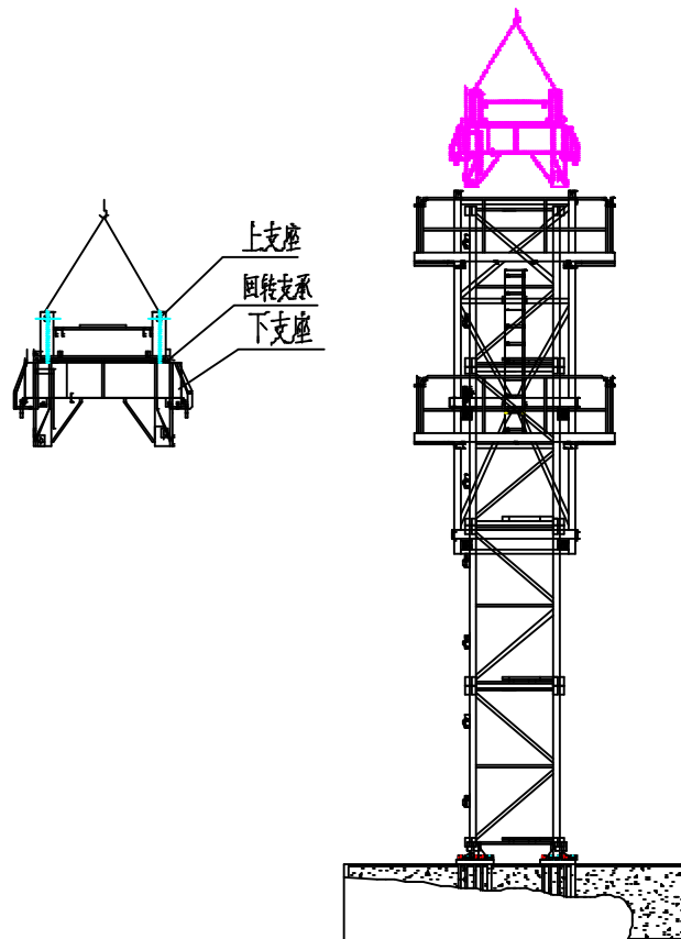
图 1.7-9 吊装回转总成
