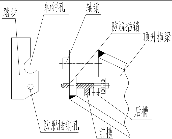
图 1.7-31 顶升防脱示意图
