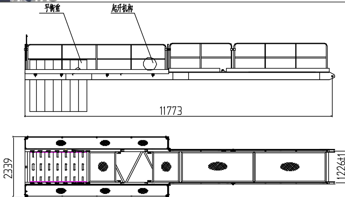
图 1.7-12 平衡臂总成
