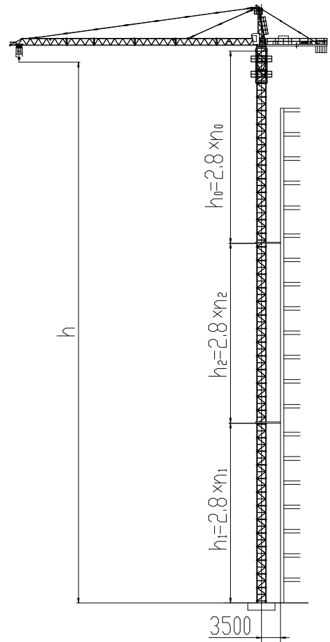
图 1.5-3 附着示意图
