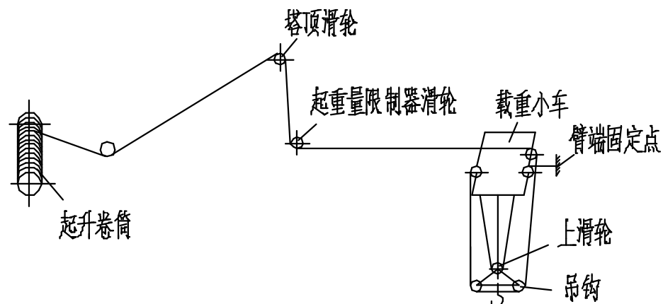
图 1.7-27 起升钢丝绳绕绳示意图
