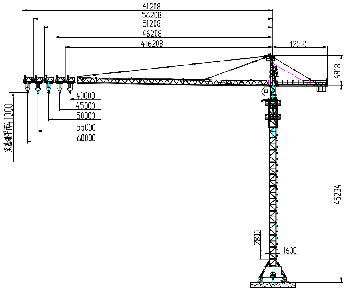
图 10.3-3 轨道行走式外形尺寸
