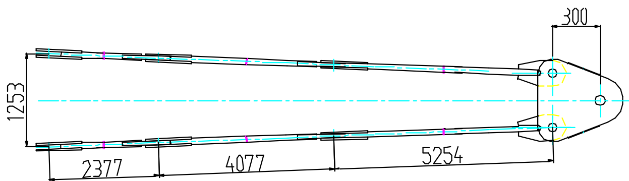
图 1.7-13 平衡臂拉杆总成
