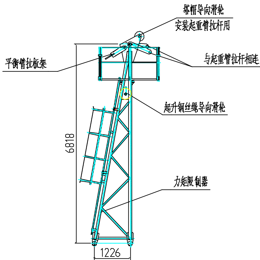
图 1.7-10 塔帽总成
