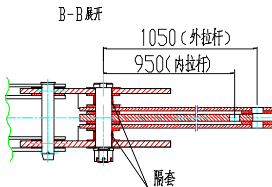
图 1.7-25 塔帽与起重臂拉杆连接处结构
