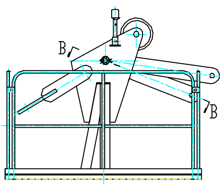
图 1.7-24 与起重臂拉杆连接处塔帽结构
