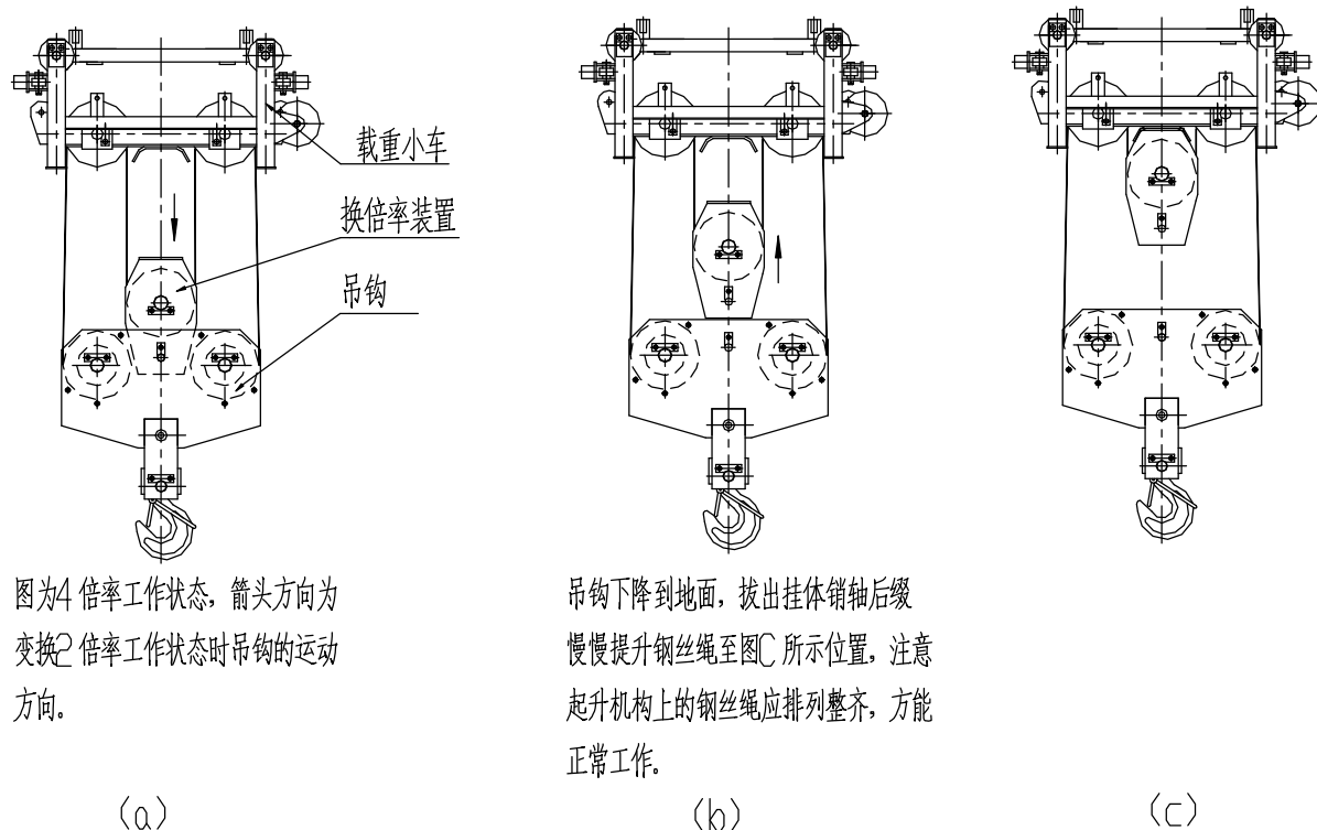
图 1.7-28 换倍率示意图
