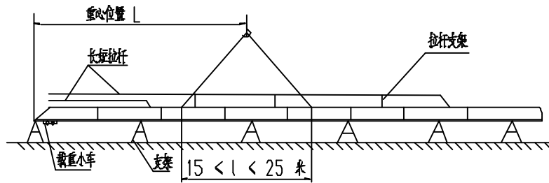
图 1.7-21 起重臂重心
