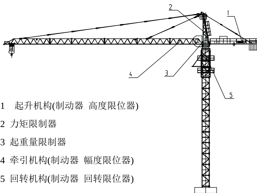
图 1.11-1 整机安全保护装置的安装位置
