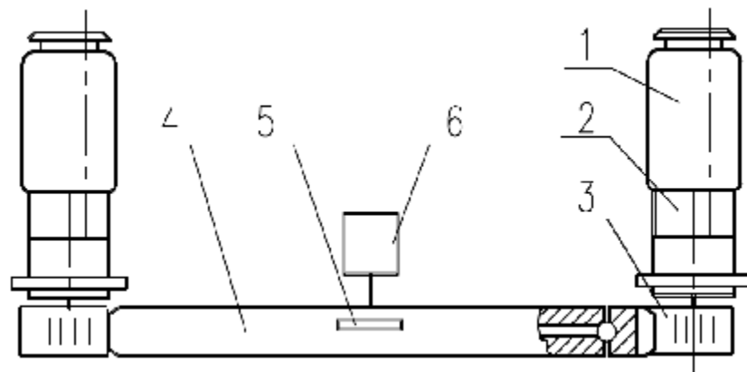
图 2.2-1 起升机构传动系统图
