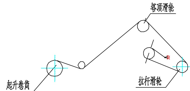
图 1.7-23 安装起重臂拉杆时起升钢丝绳绕法
