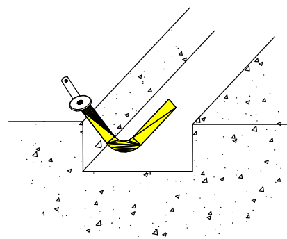
图 1.6-5C 接地装置
