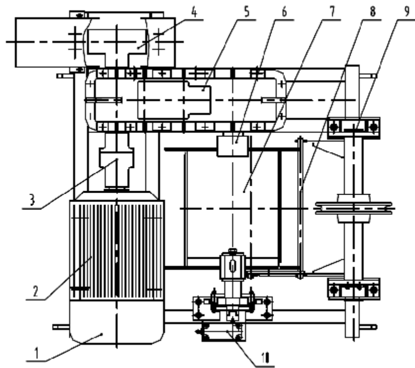
1. 电机后罩 2. 电动机 3. 联轴器 4. 制动器 5. 减速箱 6. 齿形接盘 7. 卷筒 8. 挡绳装置 9. 排绳装置 10. 高度限位器
