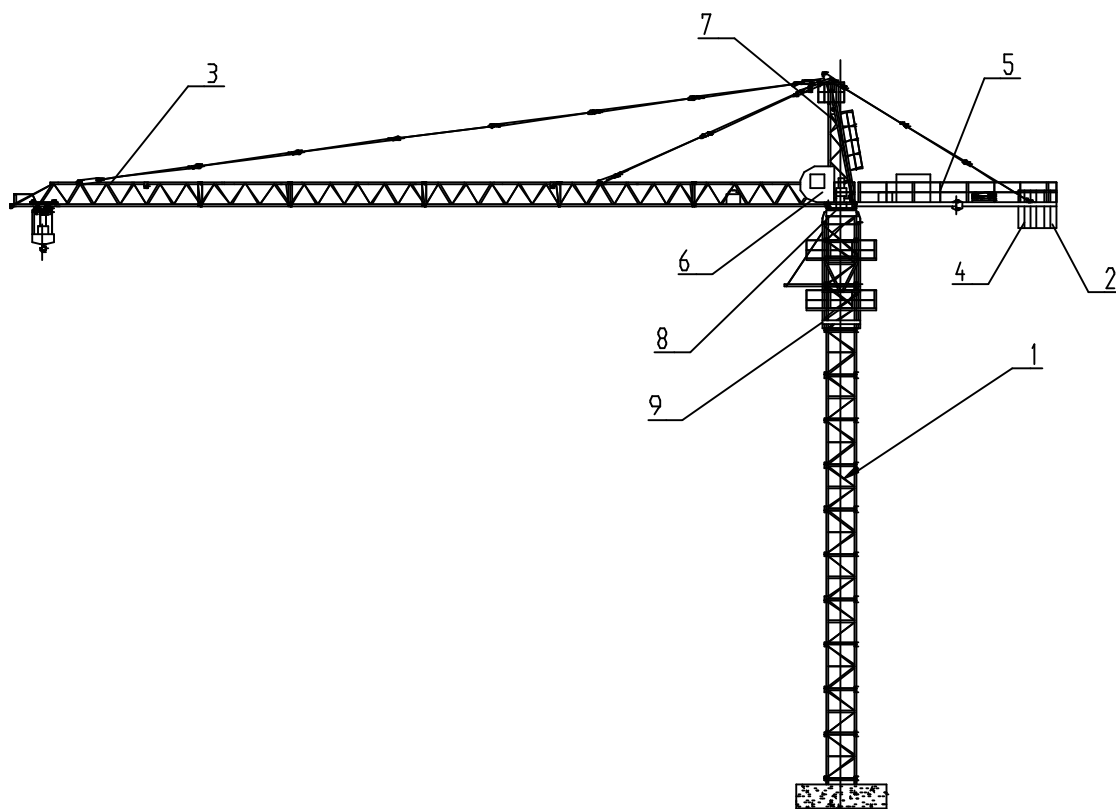
图 2.2-1 塔式起重机的拆卸
