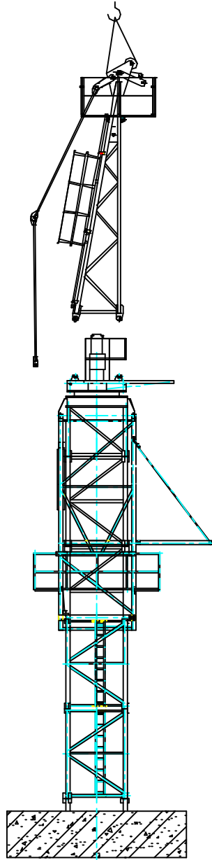
图 1.7-11 吊装塔帽总成
