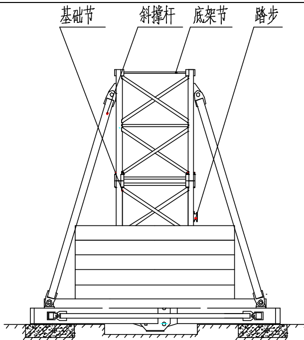
图 1.9-3 底架基础节 斜撑杆及压重的组装
