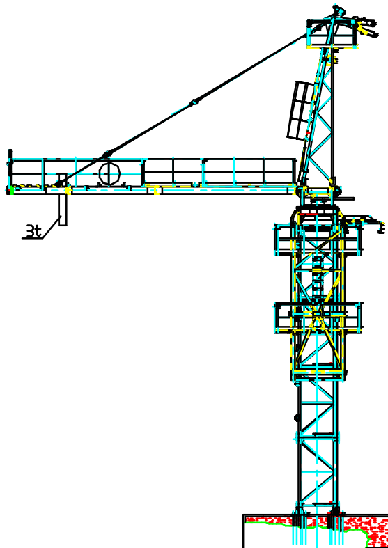
图 1.7-15 安装两块平衡重
