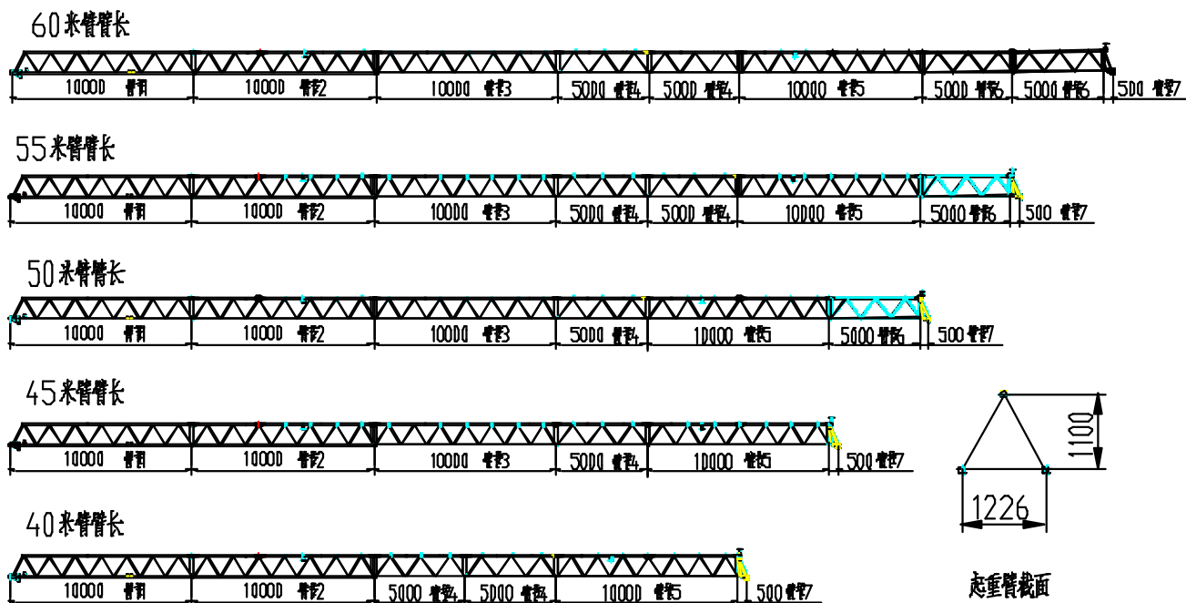
图 1.7-18 起重臂的组成
