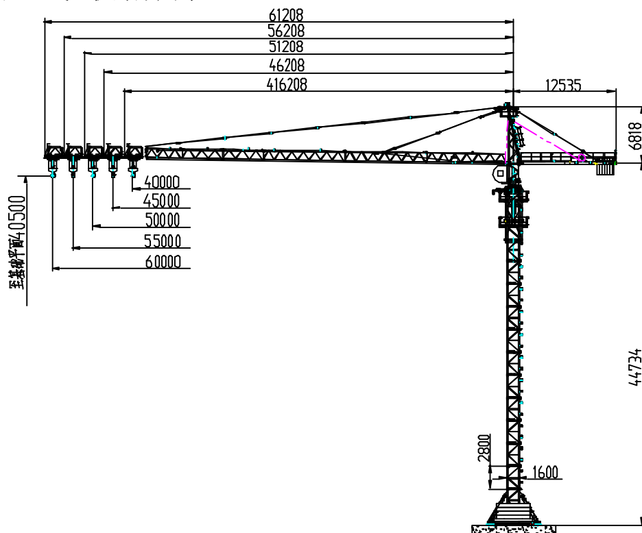
图 10.3-2 底架压重式外形尺寸
