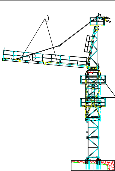
图 1.7-14 吊装平衡臂
