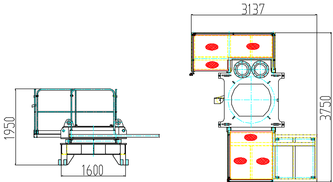
图 1.7-8 回转总成
