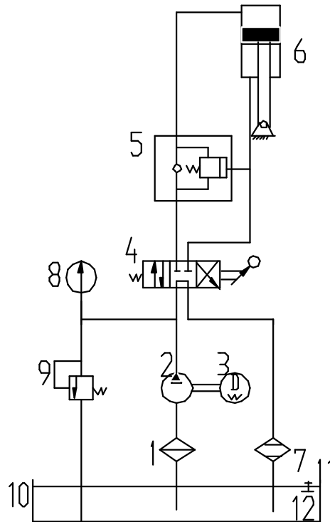
1 — 滤油器 2 — 齿轮泵 3 — 电动机 4 — 手动换向阀 5 — 平衡阀 6 — 顶升油缸 7 — 精滤油器 8 — 压力表 9 — 溢流阀 10 — 油箱 11 — 空气滤清器 12 — 滤油网
