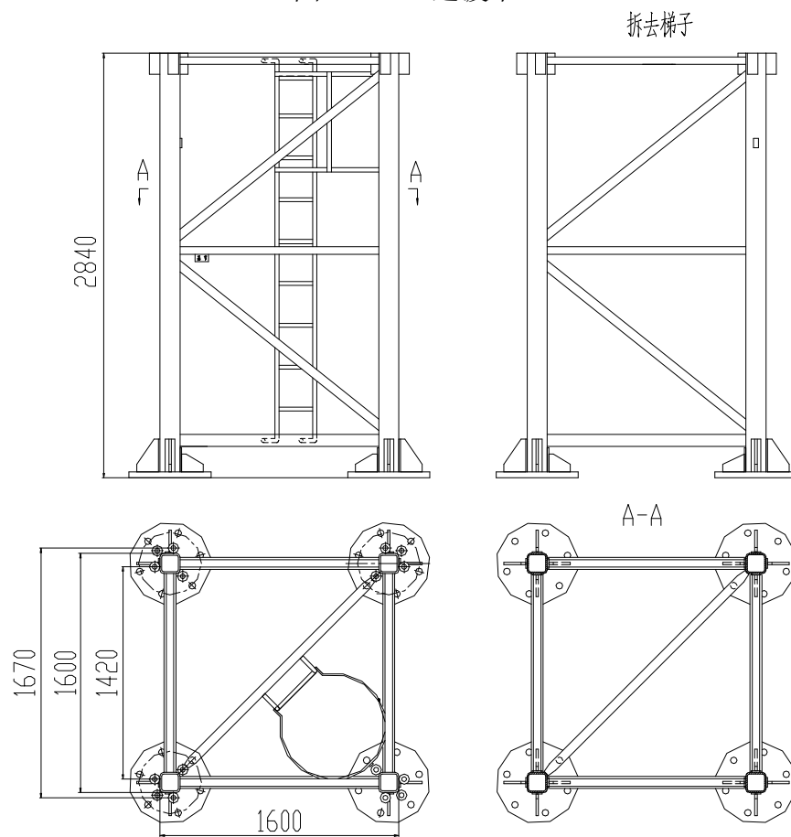
图 1.7-4 基础节
