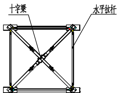
图 1.9-2 底架组装
