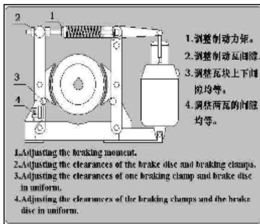
调节制动器
