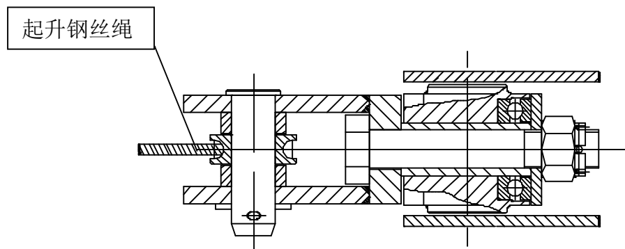
图 4.4-1 防扭装置
