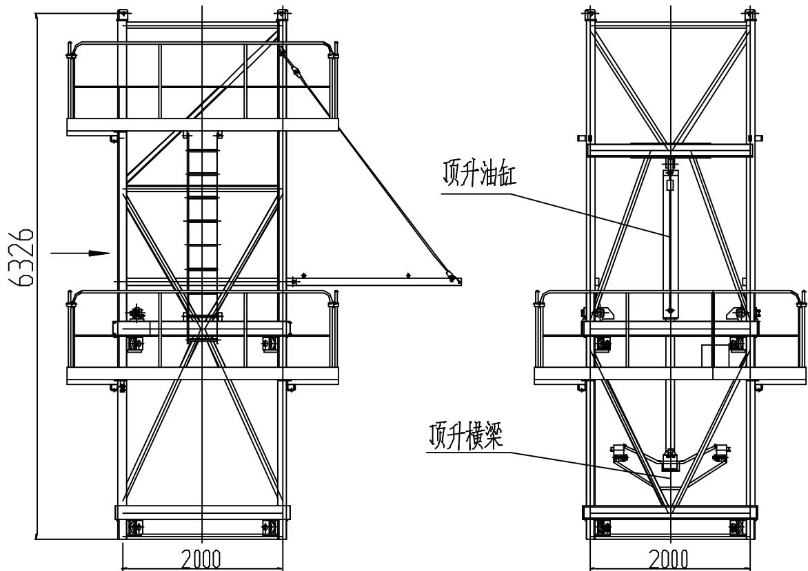
图 1.7-6 爬升架总成
