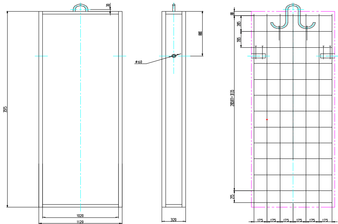
3.0t 平衡重
