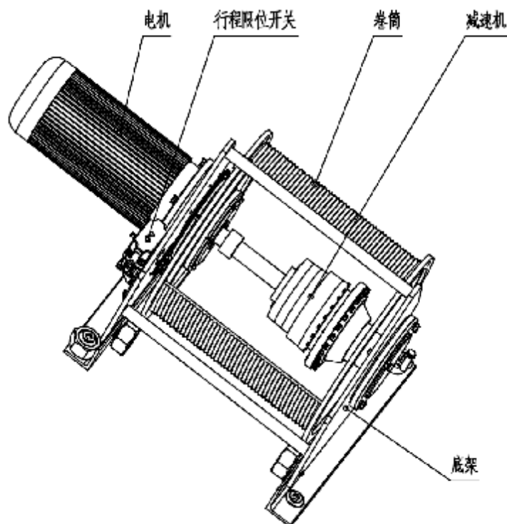
图 2.2-3 牵引机构传动系统图
