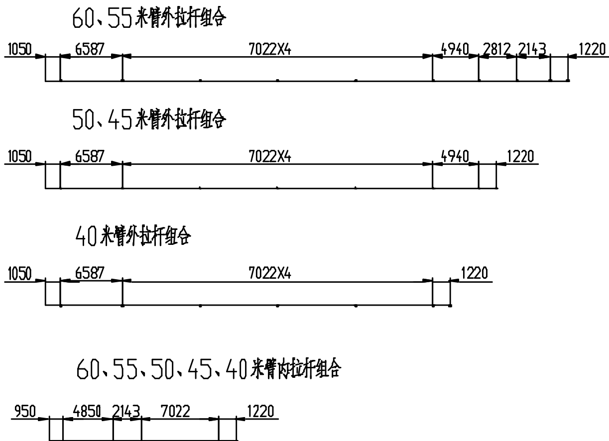
图 1.7-20 起重臂拉杆组成示意图
