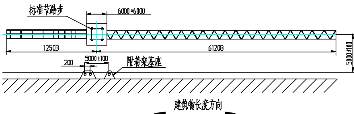
图 1.4-1 塔机安装场地的参考尺寸
