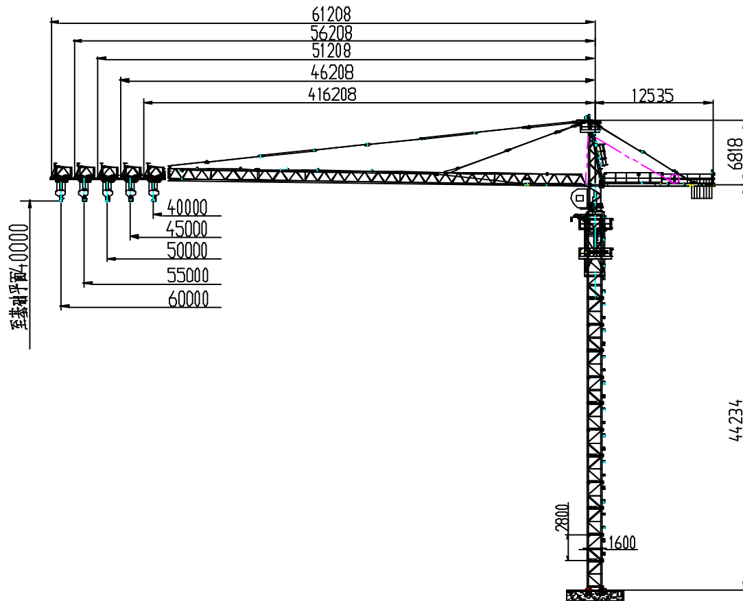
图 10.3-1 独立固定式外形尺寸
