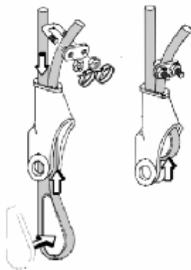
图 4.5-1 起升钢丝绳在楔套上的穿绕
