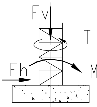
图 1.6-1 固定基础载荷示意图
