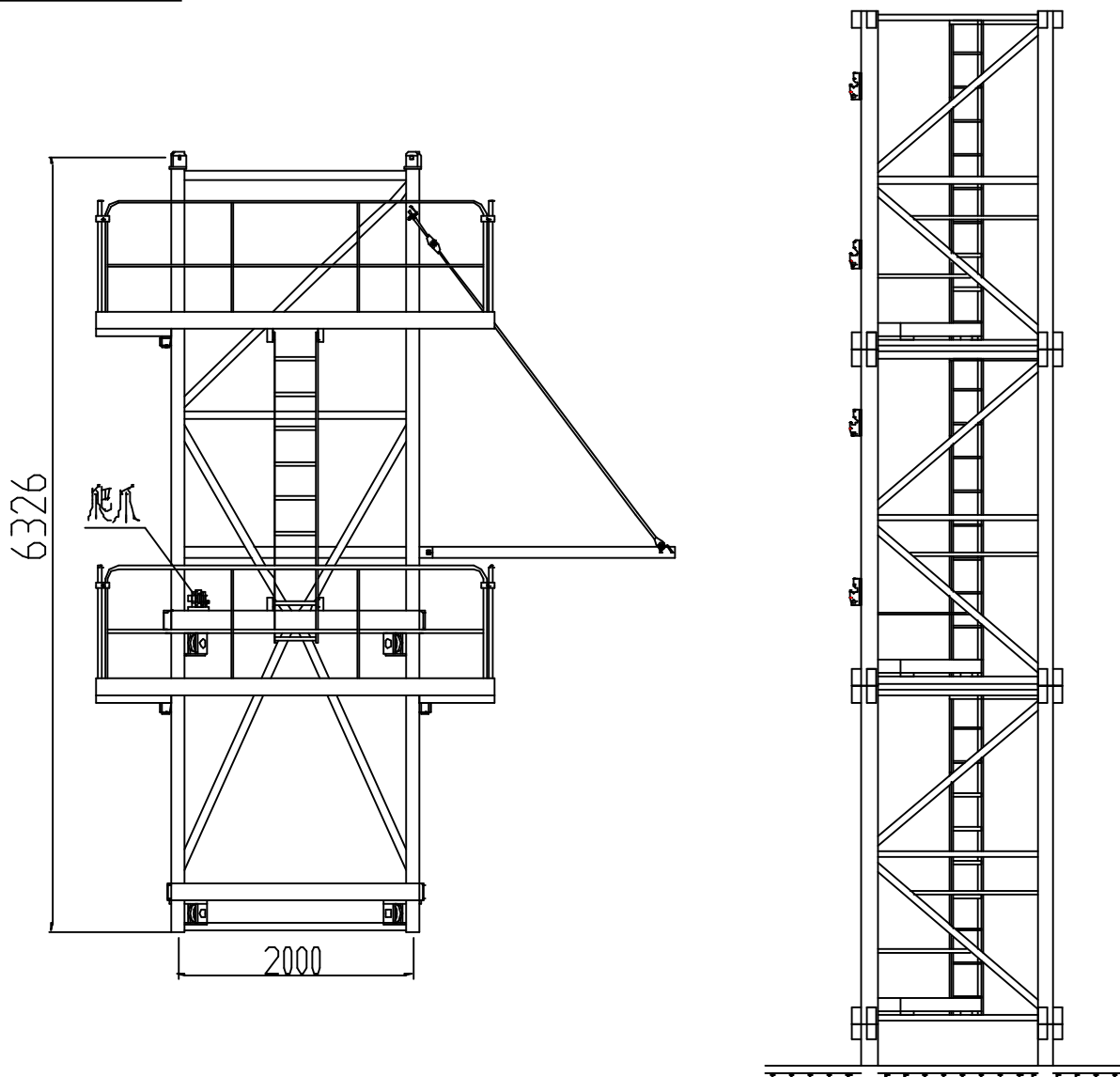
图 1.7-7 吊装爬升架
