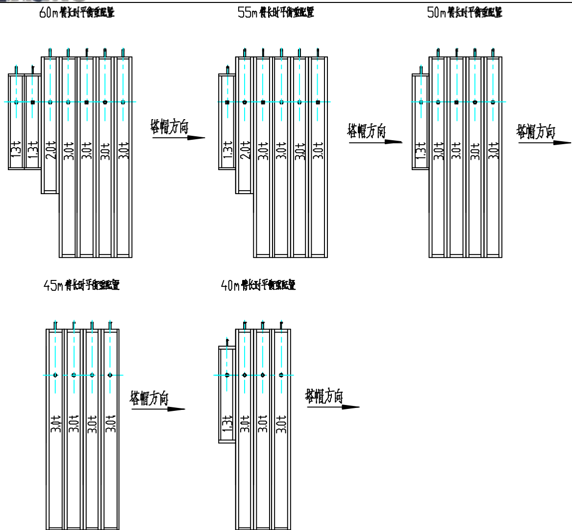
图 1.7-26 吊装平衡重
