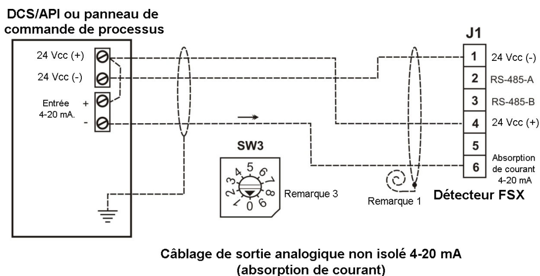
Figure 4-6 Câblage type d'une sortie analogique 4-20 mA (absorption de courant)
