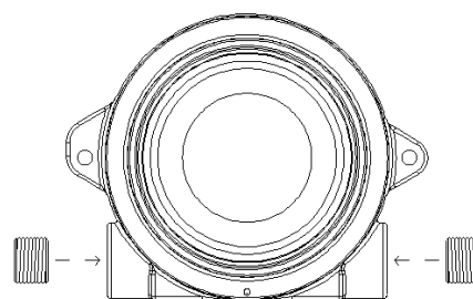
Entrées de conduit NPT ¾ po. ou 25 mm Détecteur (vue de face) Figure 2-2
