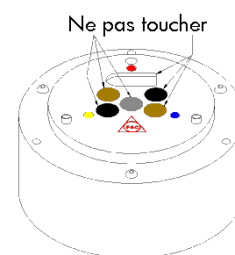
« Disque » du module de détection Figure 2-4
