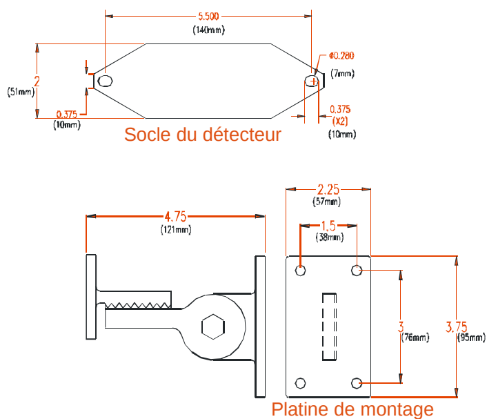
Figure 4-4 Schéma et dessins dimensionnels pour SM4
