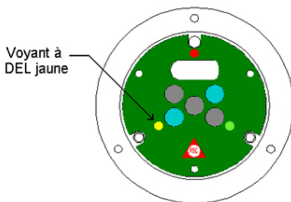
Figure 3-5 Module de détection, vue de face
