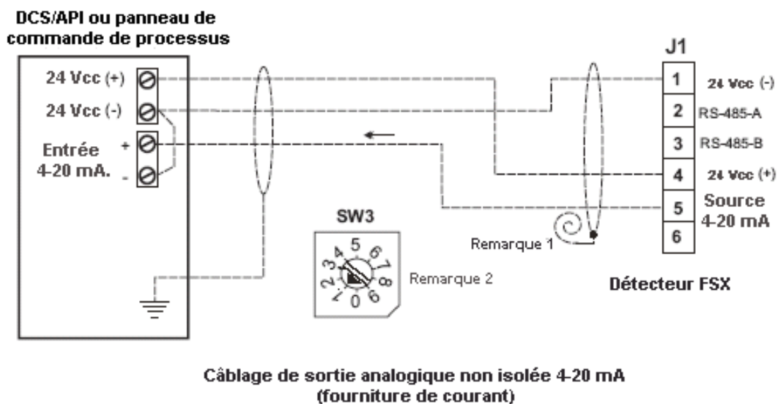
Figure 4-5 Câblage type d'une sortie analogique 4-20 mA (fourniture de courant)
