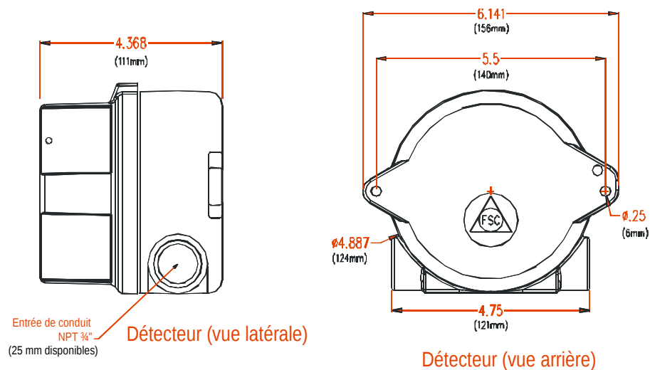
Figure 4-3 Schéma et dessins dimensionnels pour FS19X/FS20X
