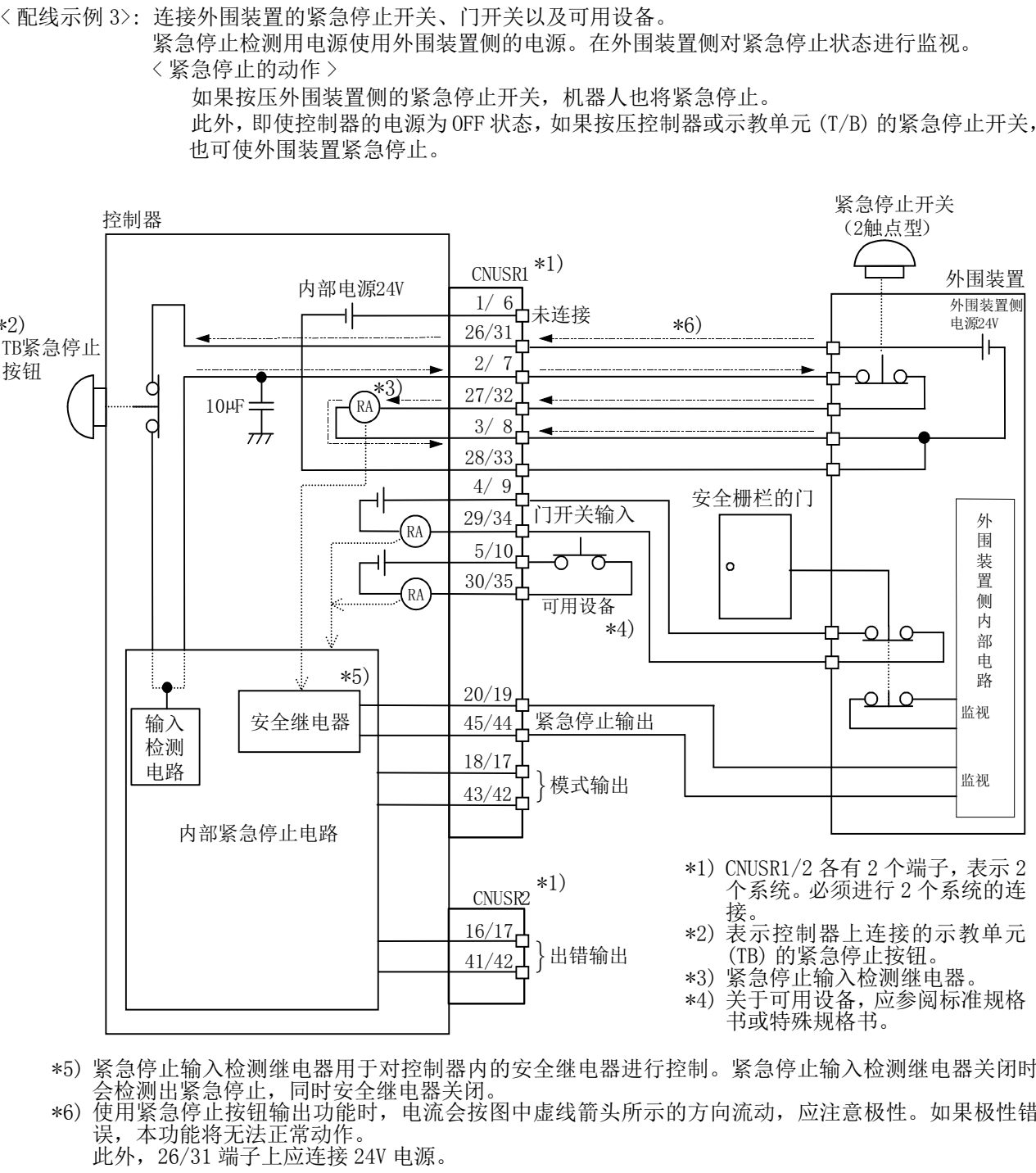
图 6-3：安全措施示例 (CR751 配线示例 3)
