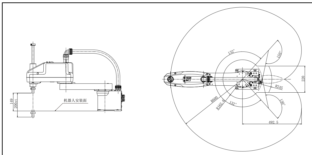
图 2-13: RH-6CH6020-S11 动作范围图
