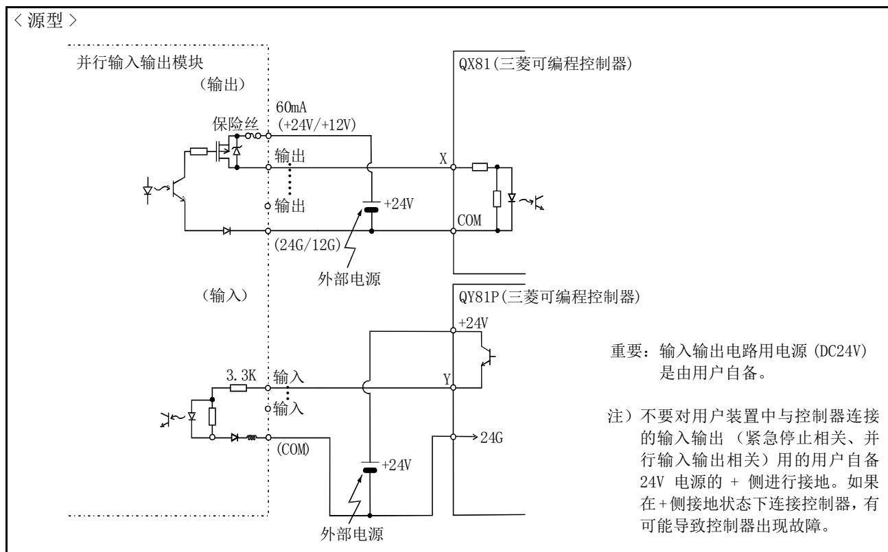
图 3-24：与三菱可编程控制器的连接示例（源型）
