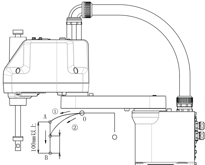
图 2-8：在 Z 轴最下端进行定位时的推荐路径
