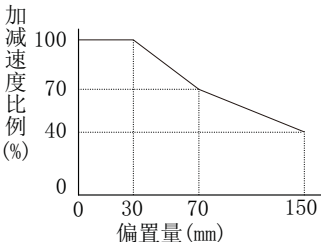
图 2-6：偏置量和最大速度的关系
