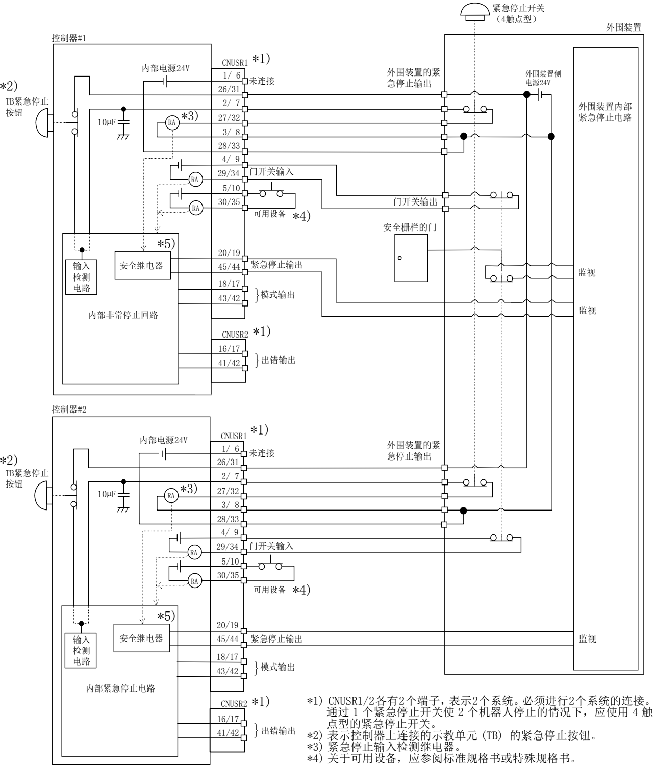
图 6-4：安全措施示例 (CR751 配线示例 4)
