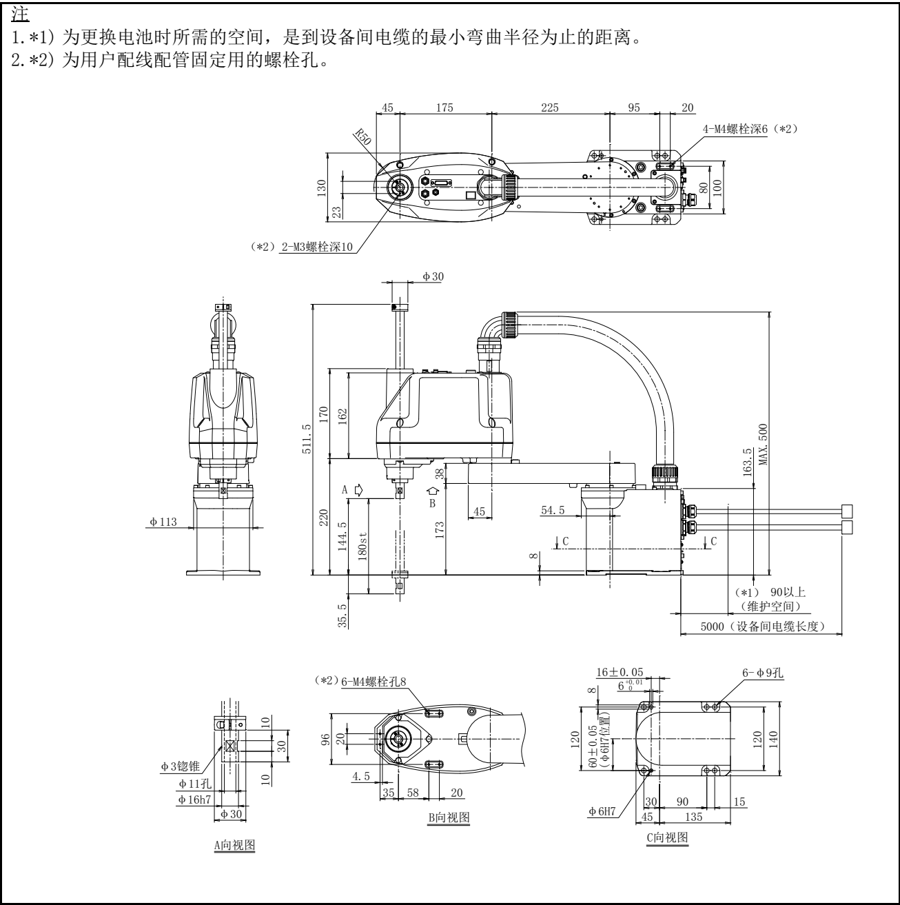
图 2-10：RH-3CH4018-S11 本体外形图
