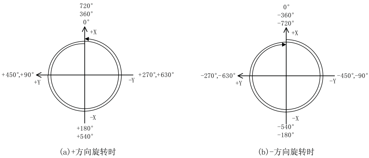
图 4-2：RH-3CH-S11/RH-6CH-S11 的 C 成分的定义（超出 \pm 180^\circ 显示）
