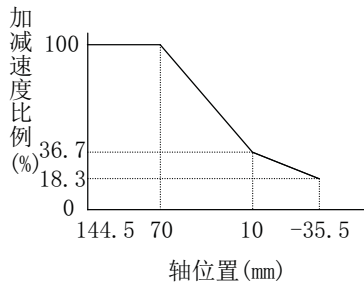
RH-3CH-S11 J3 轴 (Z) 行程 180mm (标准加减速速度)
