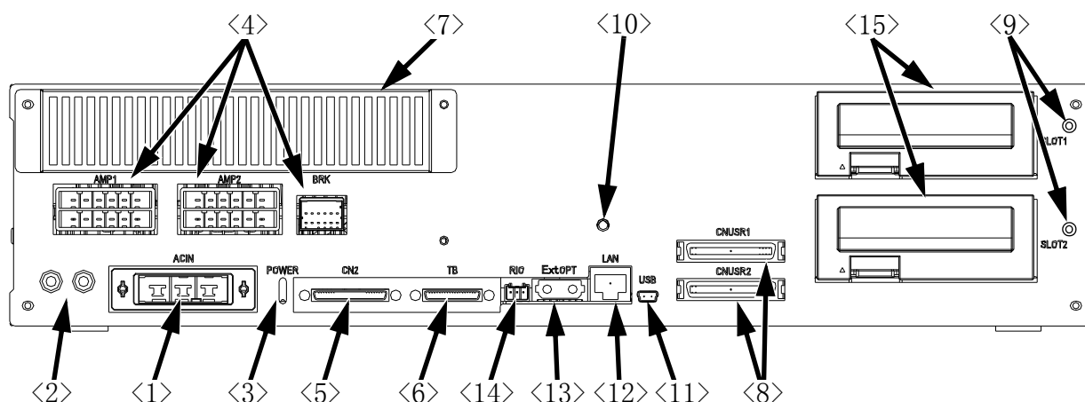
控制器背面
