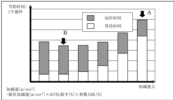
图 2-7：加减速度和节拍时间的关系（示意图）
