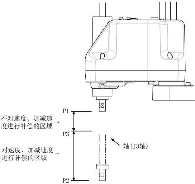
图 2-4: 加减速度的补偿区域
