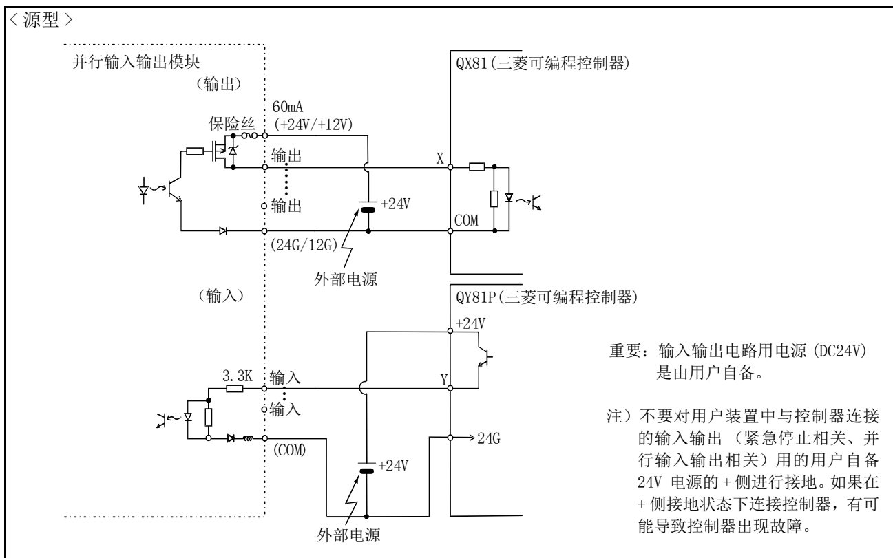
图 3-31：与三菱可编程控制器的连接示例（漏型）
