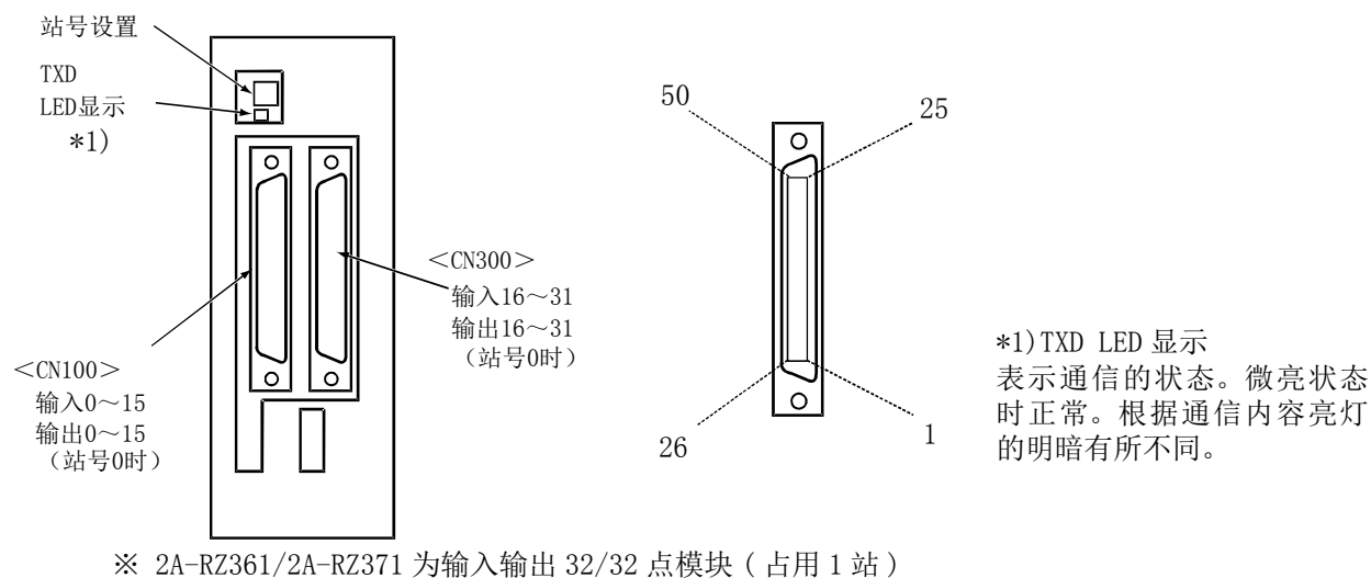
图 3-29：并行输入输出模块的连接器针配置
