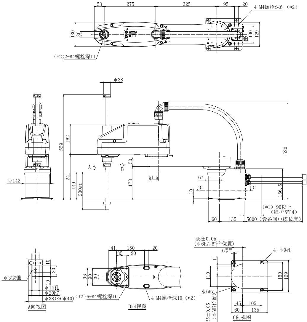
图 2-12: RH-6CH6020-S11 本体外形图
