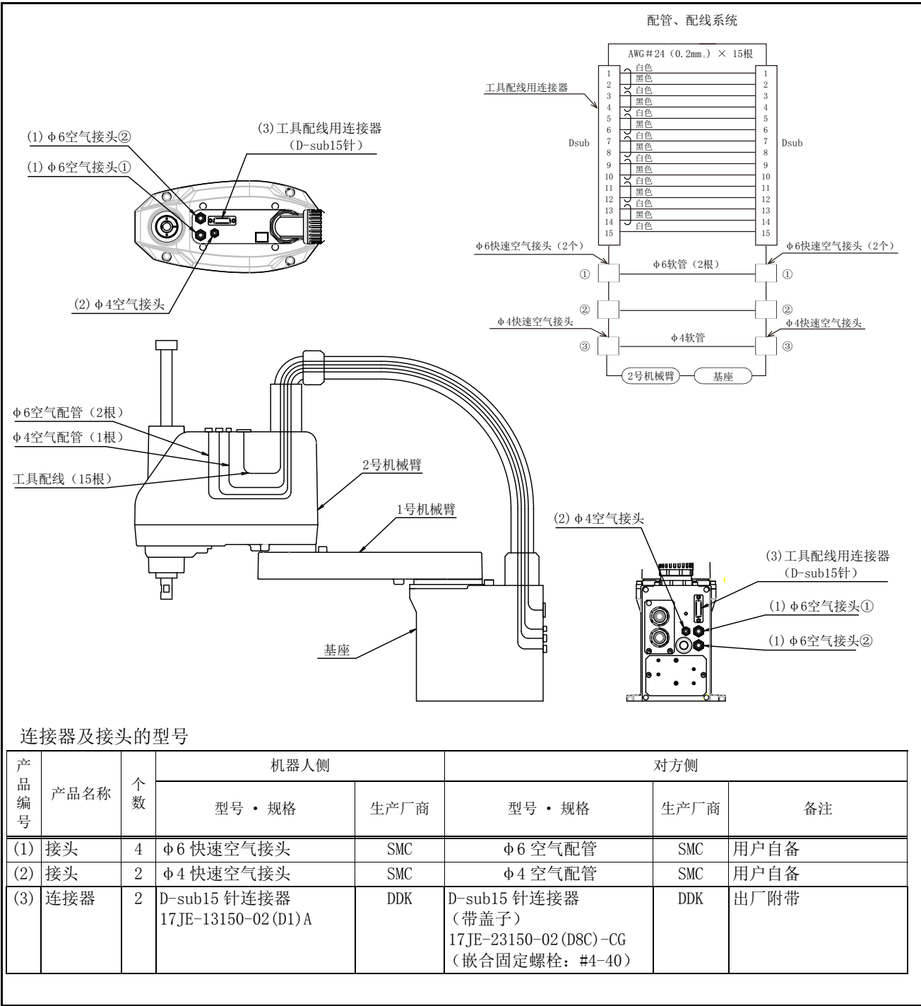
图 2-16: 抓手用配线・配管
