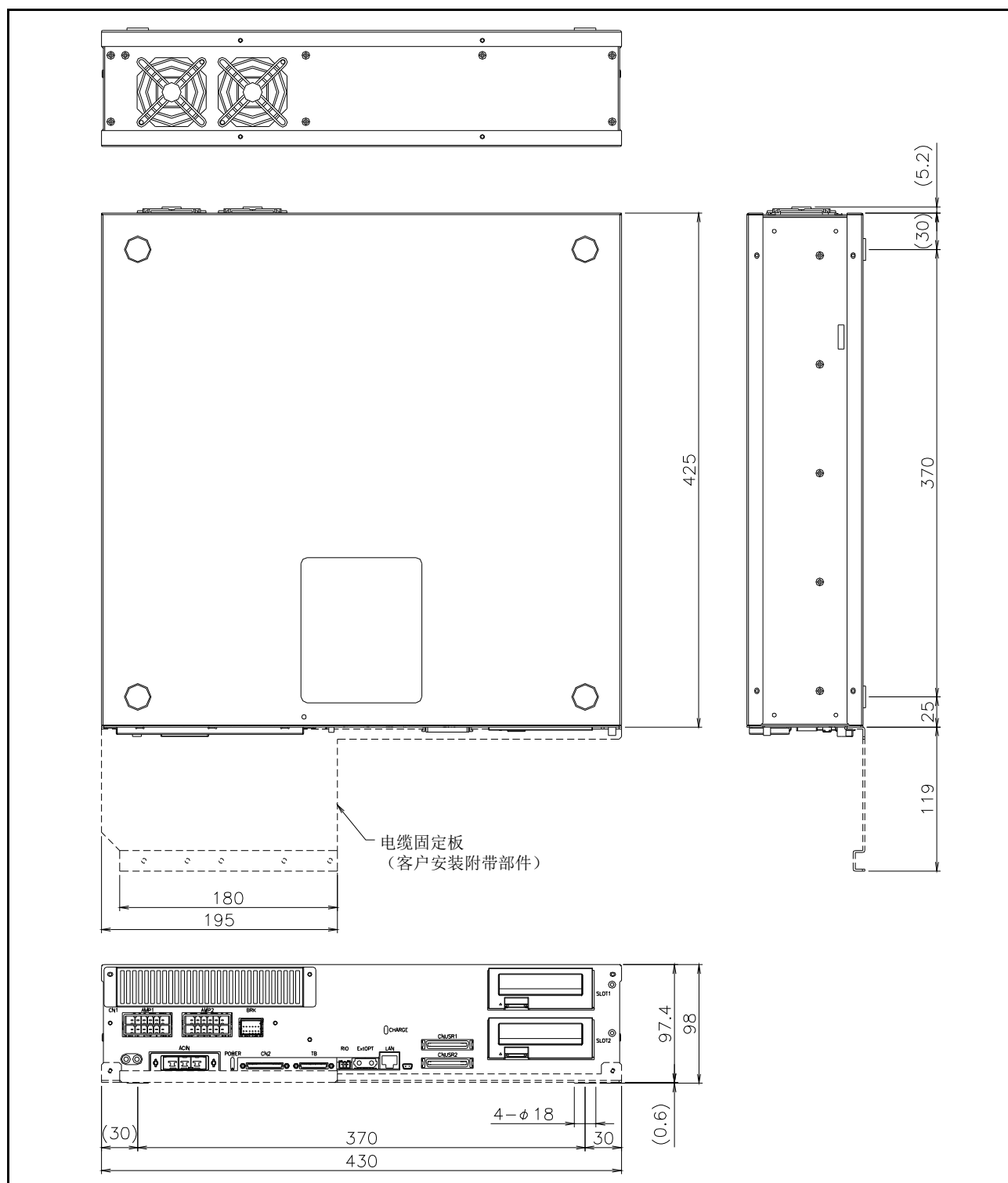
图 3-2: 控制器的外形尺寸图 (CR751)
