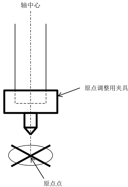
图 4-3：原点调整
