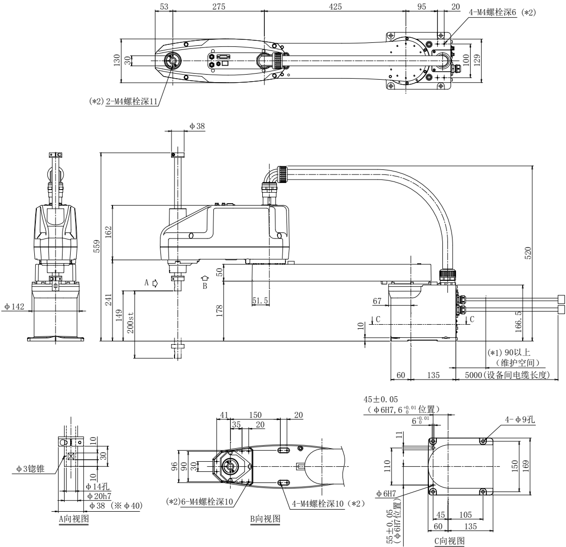
图 2-14: RH-6CH7020-S11 本体外形图
