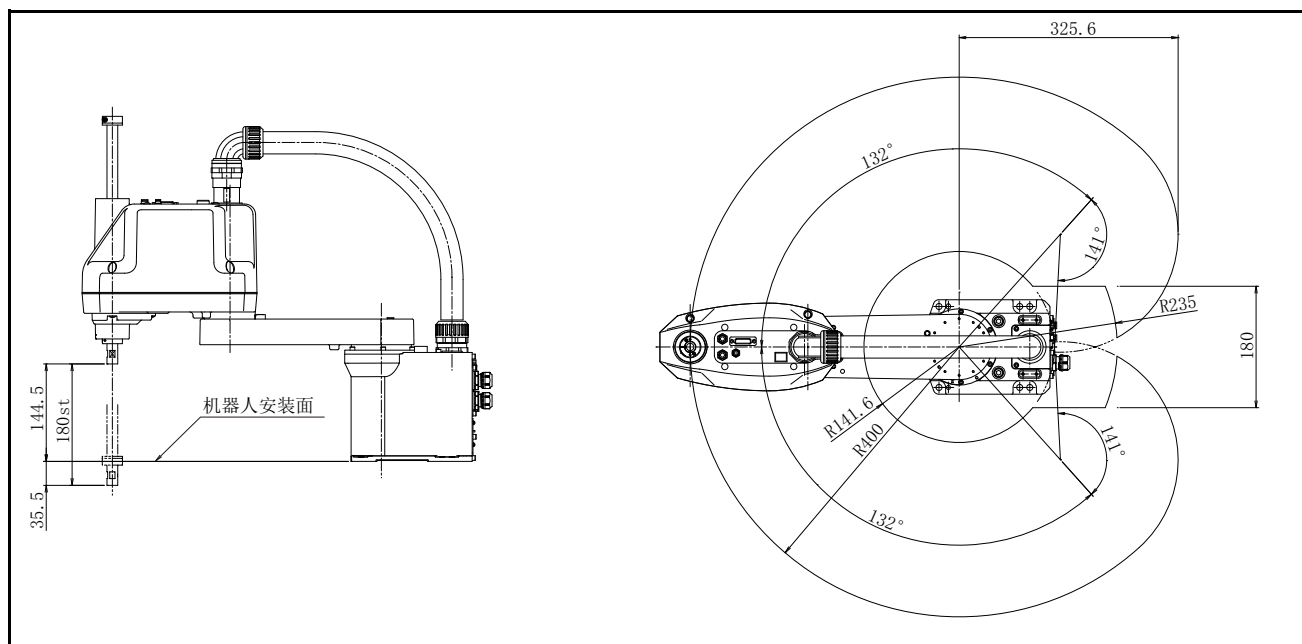
图 2-11: RH-3CH4018-S11 动作范围图
