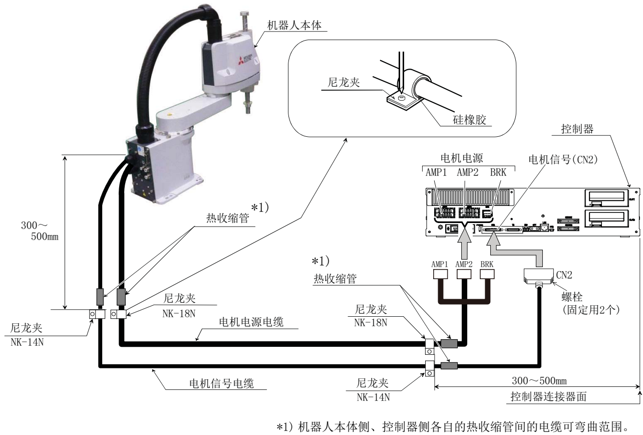
图 2-19：弯曲用电线的固定方法
