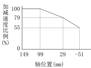
图 2-5：加减速速度的自动补偿
