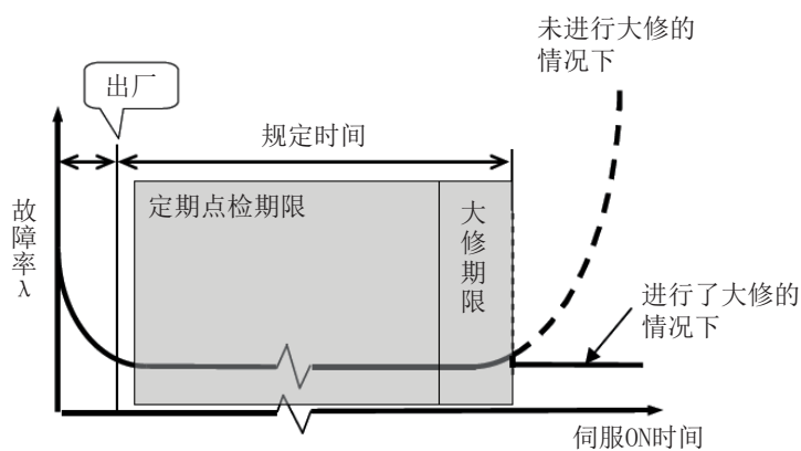
图 2-20: 定期点检期限・大修时间
