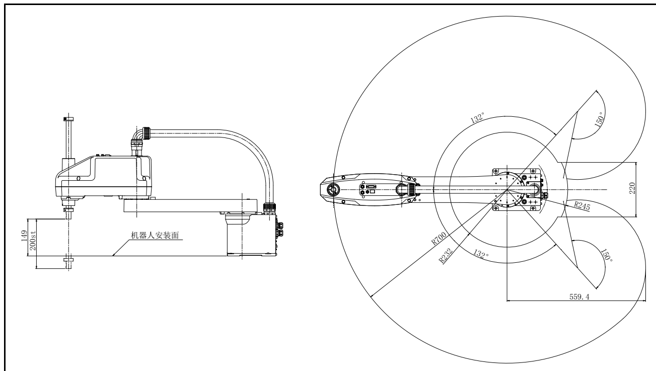
图 2-15: RH-6CH7020-S11 动作范围图
