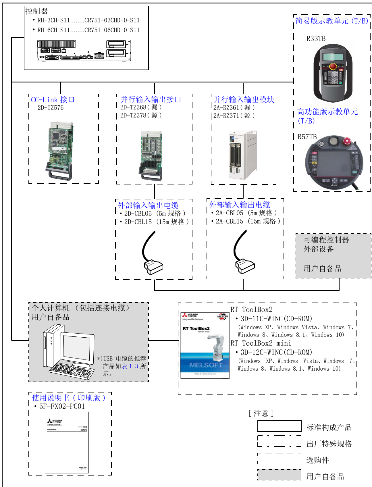
图 1-2：构成设备的概要（控制器）
