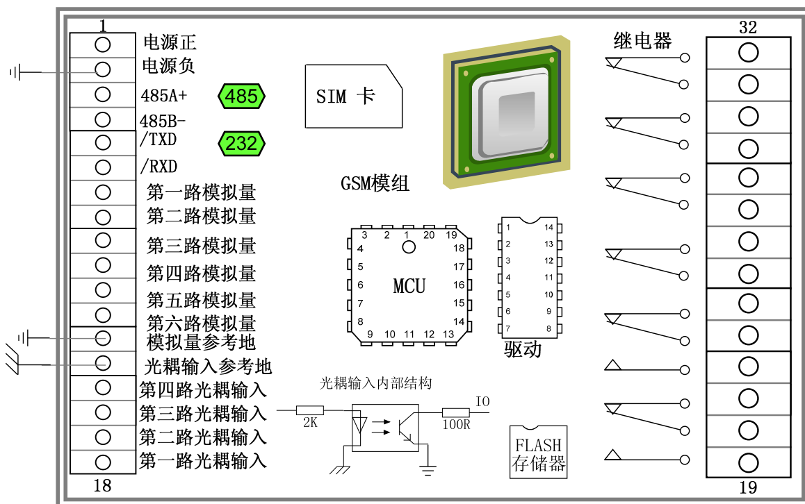
图 1-3 RTU6640 内部功能结构图
