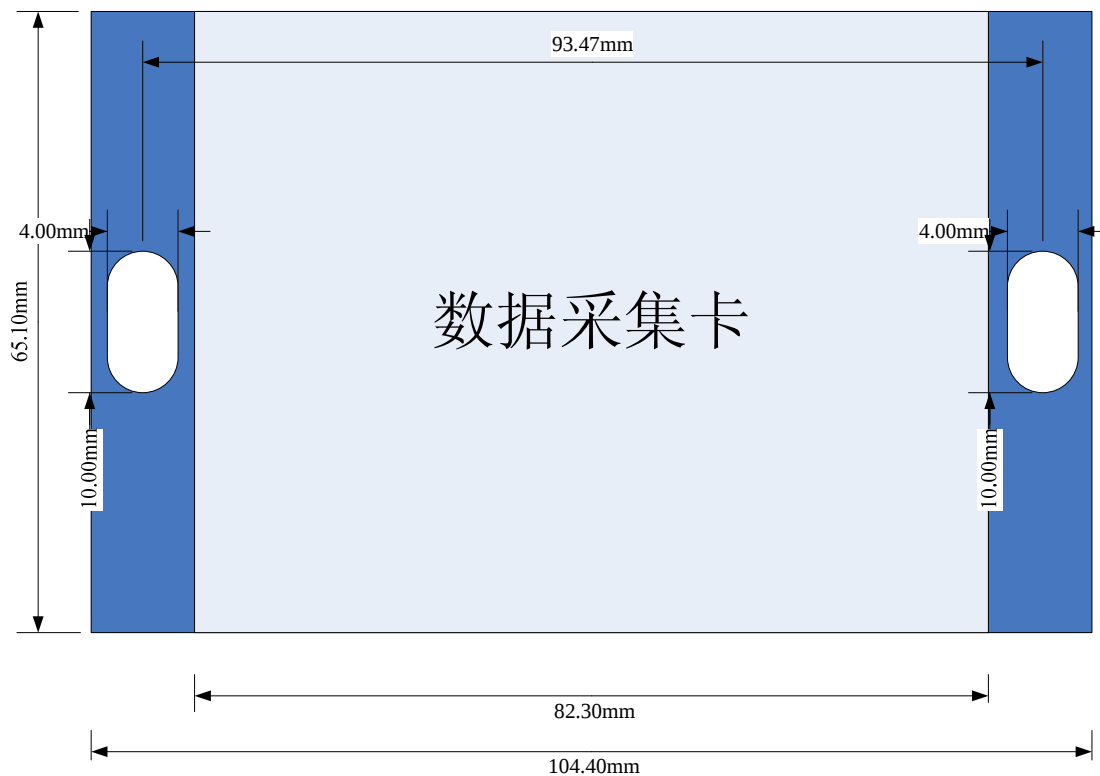
图 1-1 机械结构图
