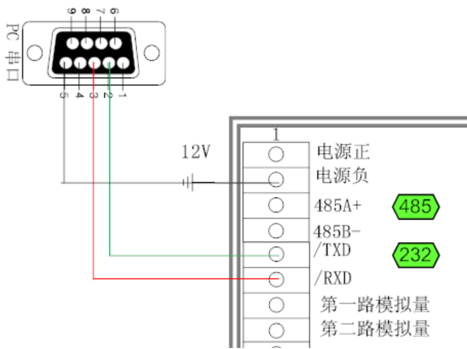
图 1-4 RTU4100 通讯接口结构图
