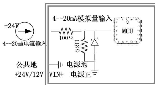
图 1-5 RTU4100 4-20mA 模拟量输入内部结构图 如果购买的是 4-20mA 或 0-20mA 模式
