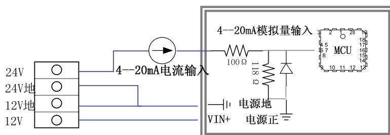
图 1-5 RTU4100 4-20mA 模拟量接入方式
