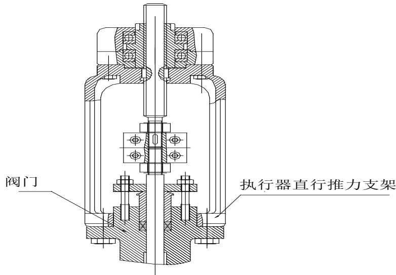
图 6-2 RQIV003~RQIV060、RQMIV03~RQMIV54 型执行机构丝杠与阀门连接形式示意图
