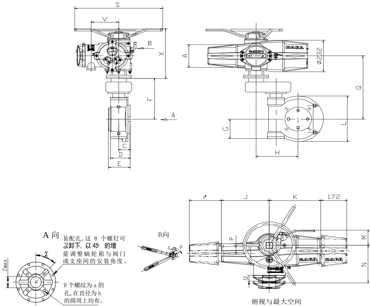
图 6-7 RGD/RGW 蜗轮箱与带二级减速执行机构组合尺寸图
