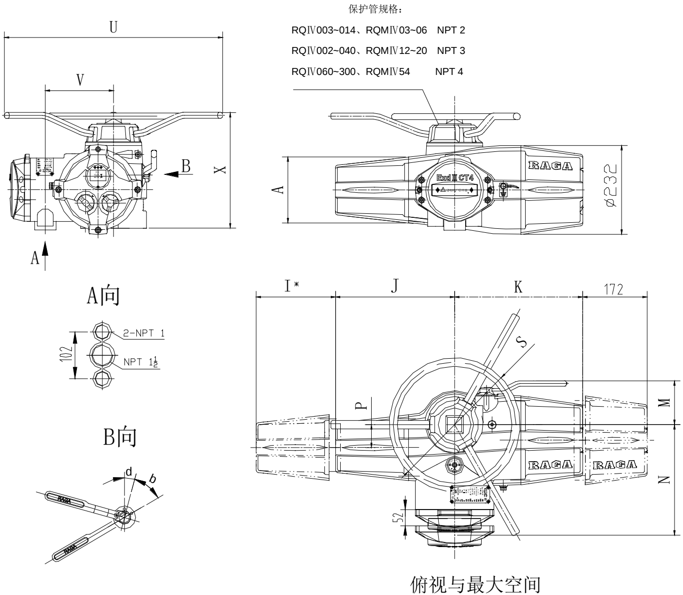
图 6-4 RQIV003~ RQIV100、RQMIV型执行机构安装尺寸图
