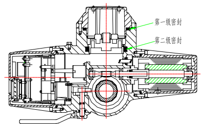
图 3-2 双密封结构
