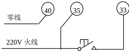
外部供电“有信关,无信开”外部接线
