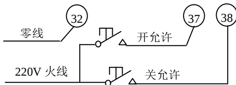
外部供电：开阀联锁和关阀联锁外部接线
