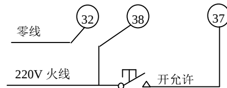
外部供电：仅开阀联锁外部接线
