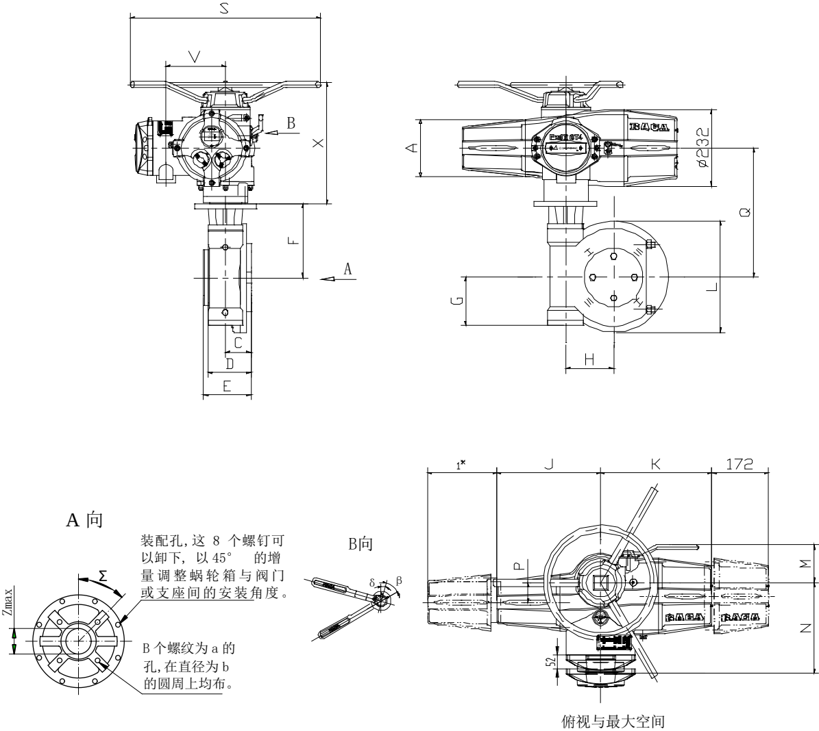
图 6-6 RGD/RGW 蜗轮箱与执行机构组合尺寸图
