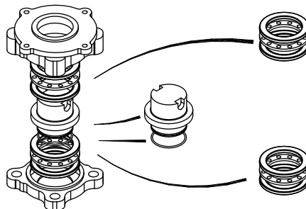
图 6-1 RQIV003~RQIV060、RQMIV03~RQMIV54 型执行机构与 A 型驱动套连接形式示意图
