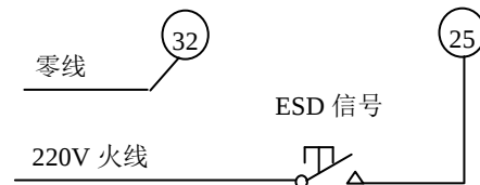
外部供电：ESD 控制外部接线
