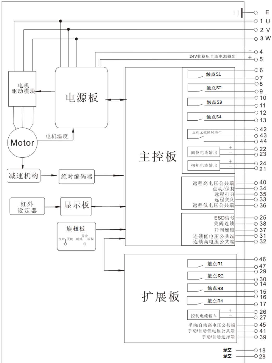
AGA 多回转电动执行器内部结构和连线图
