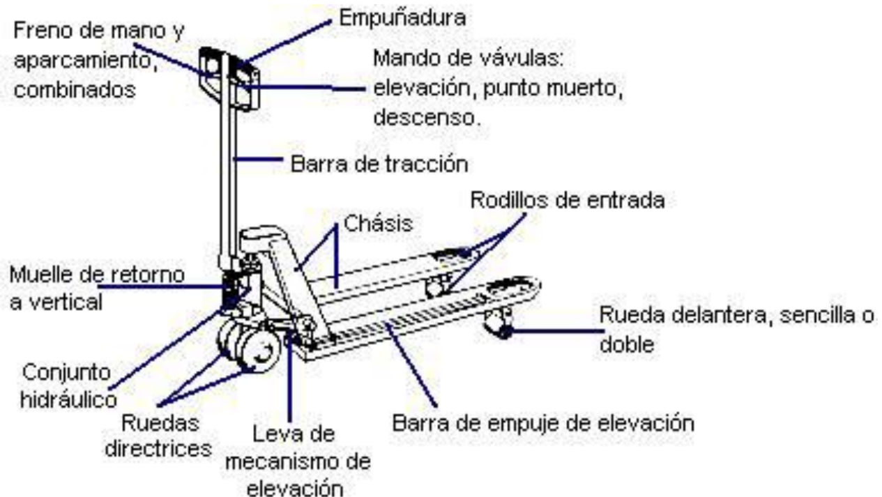
Figura 1. Partes principales del estibador manual.
