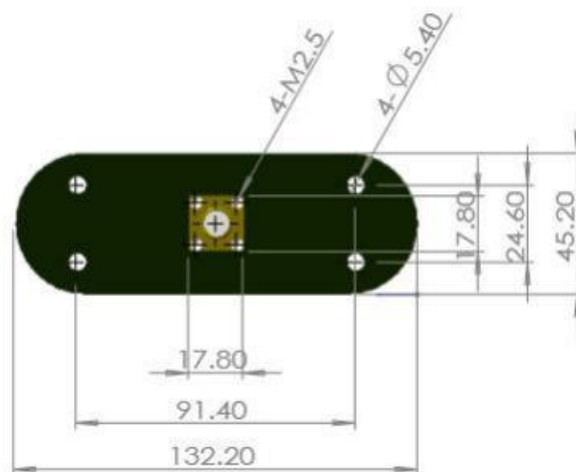
设备外廓尺寸和安装形式
