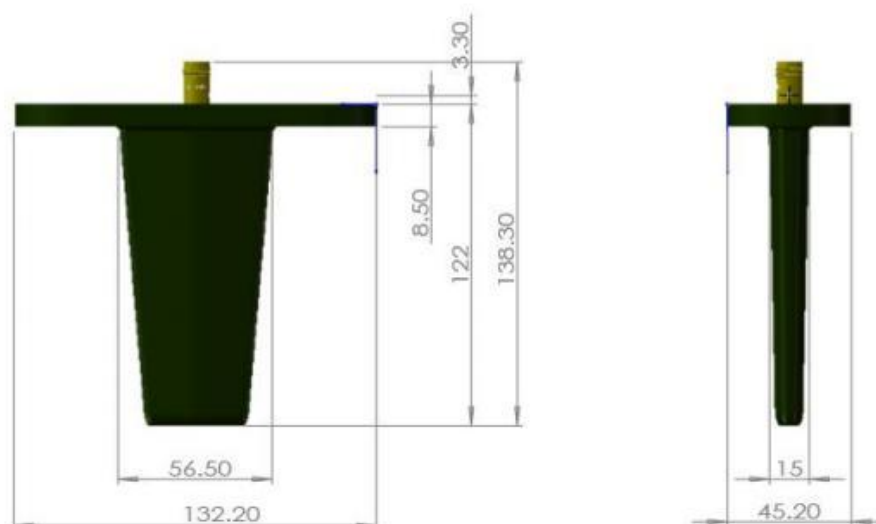
天线外廓尺寸
