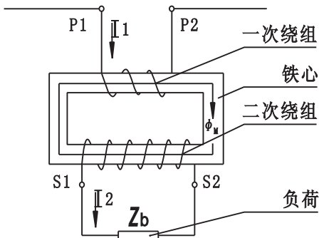
电流互感器工作原理图
