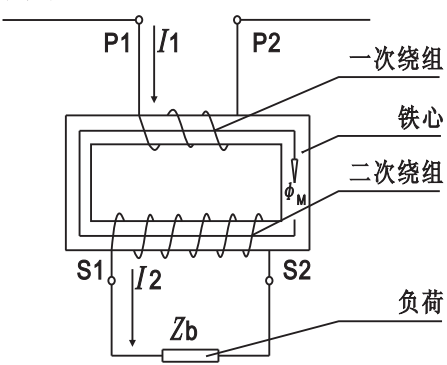
电流互感器工作原理图
