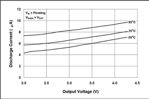
图 2-7: 输出反向漏电流—输出电压关系曲线
