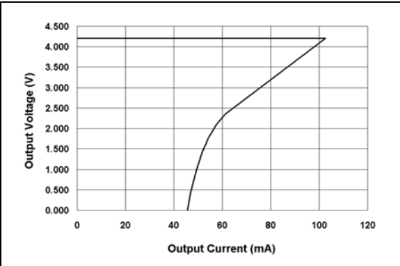
图 2-9: 监听限流曲线
