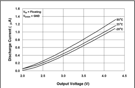
图 2-8: 输出反向漏电流—输出电压关系曲线
