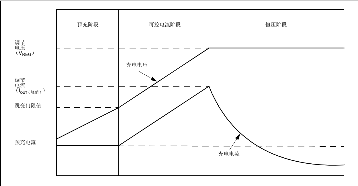
图 6-2：典型充电曲线
