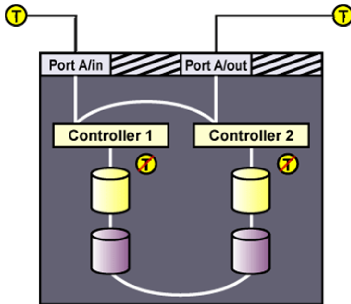
连接到多后始端 SCSI 总线的双控制器 RAID 阵列
