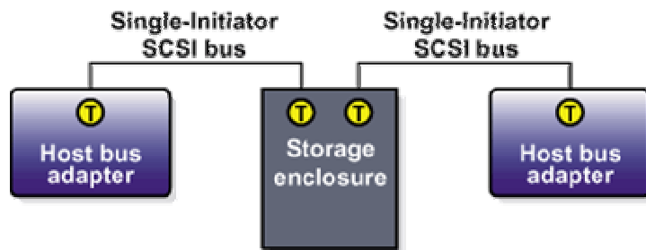
单启始端 SCSI 总线配置
