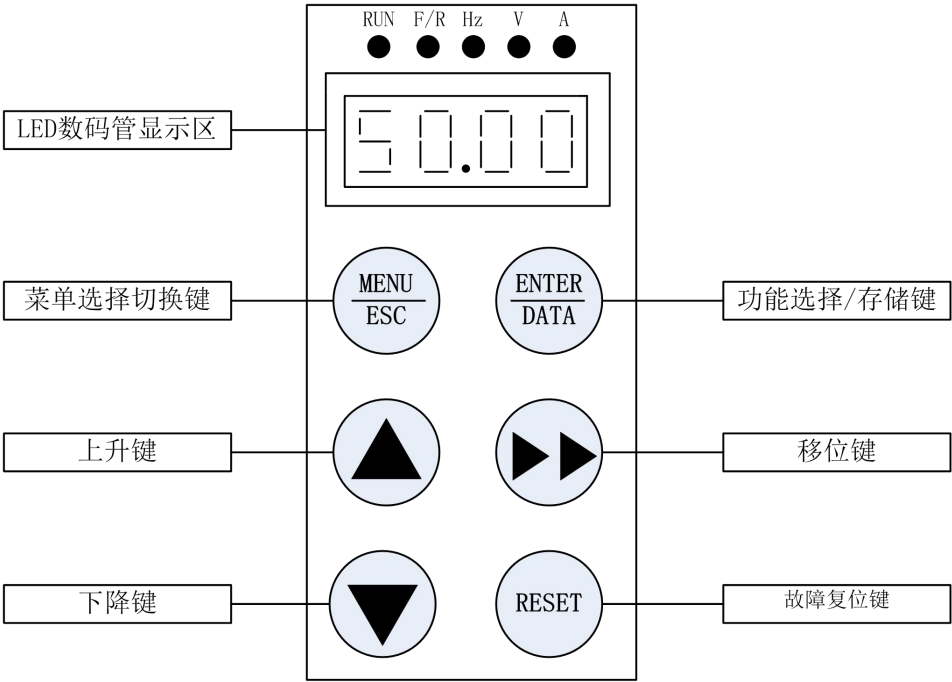
图3-1 操作面板（键盘）示意图
