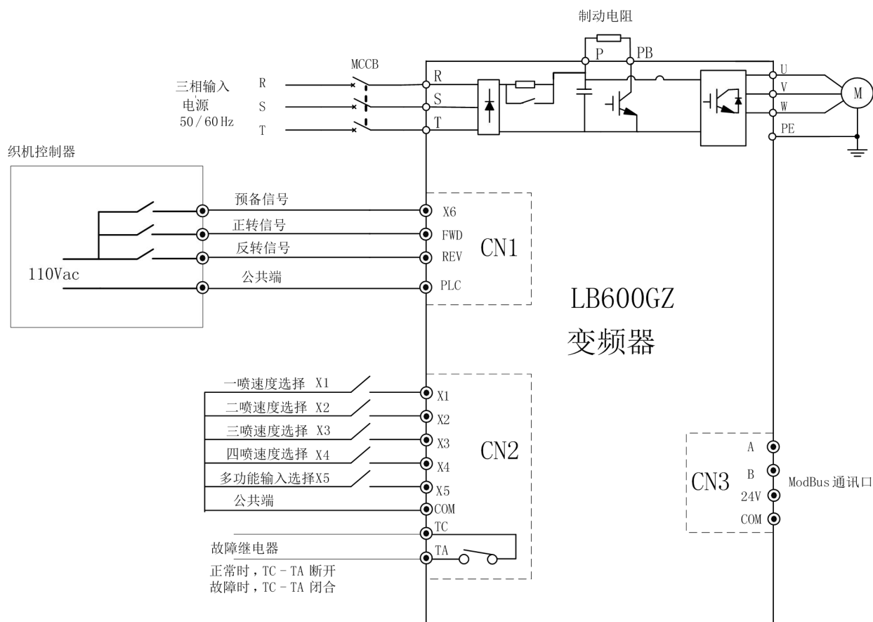
图 2-1 LB600GZ 变频器基本配线图
