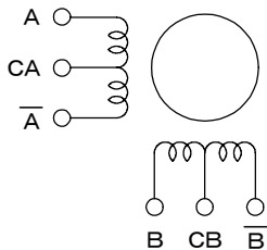
Motor Wiring
