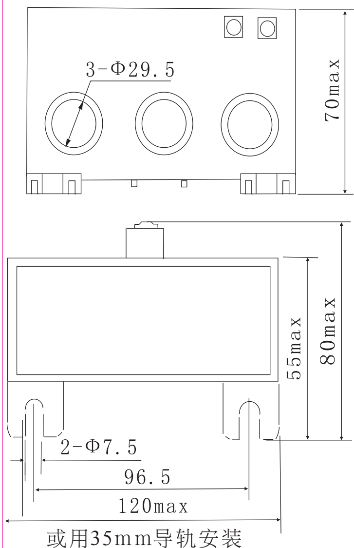
64A-160A 128A-320A 外形及安装尺寸图
