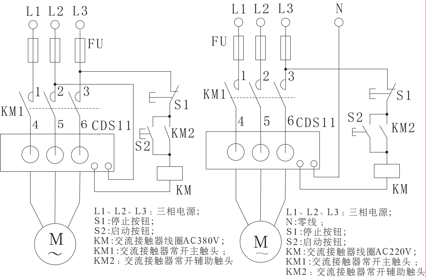
应用电路接线举例
