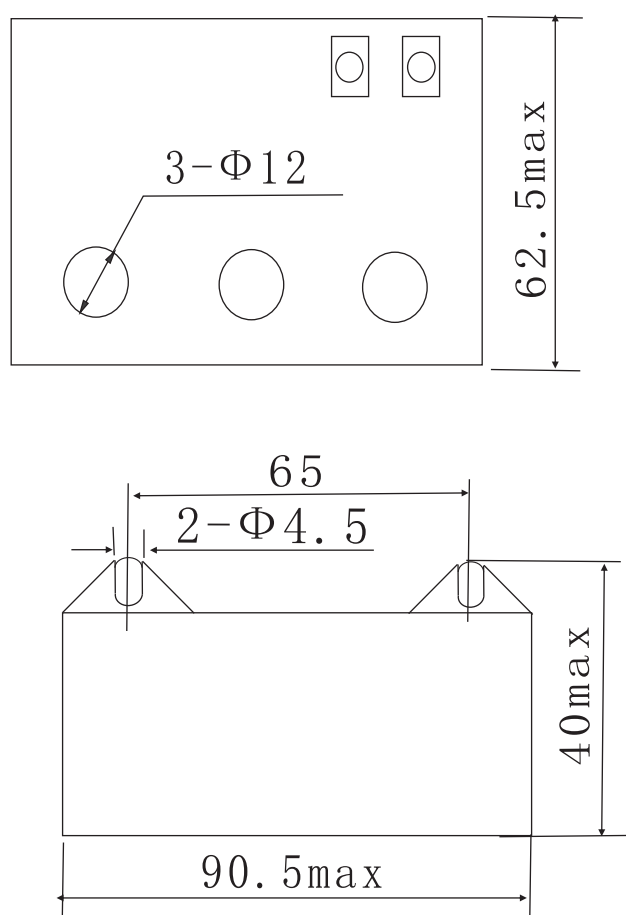
2.5-80A外形及安装尺寸图
