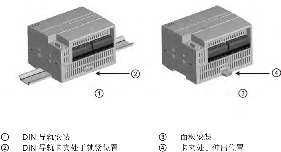
图 3-1 在 DIN 导轨或面板上安装
