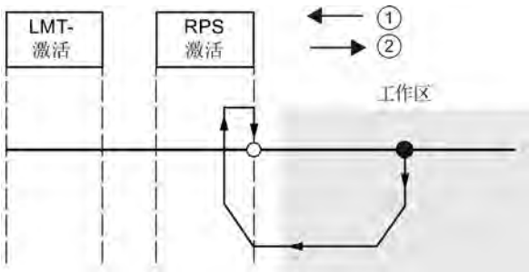
图 12-1 ①: RP 搜索方向 ②: RP 接近方向
