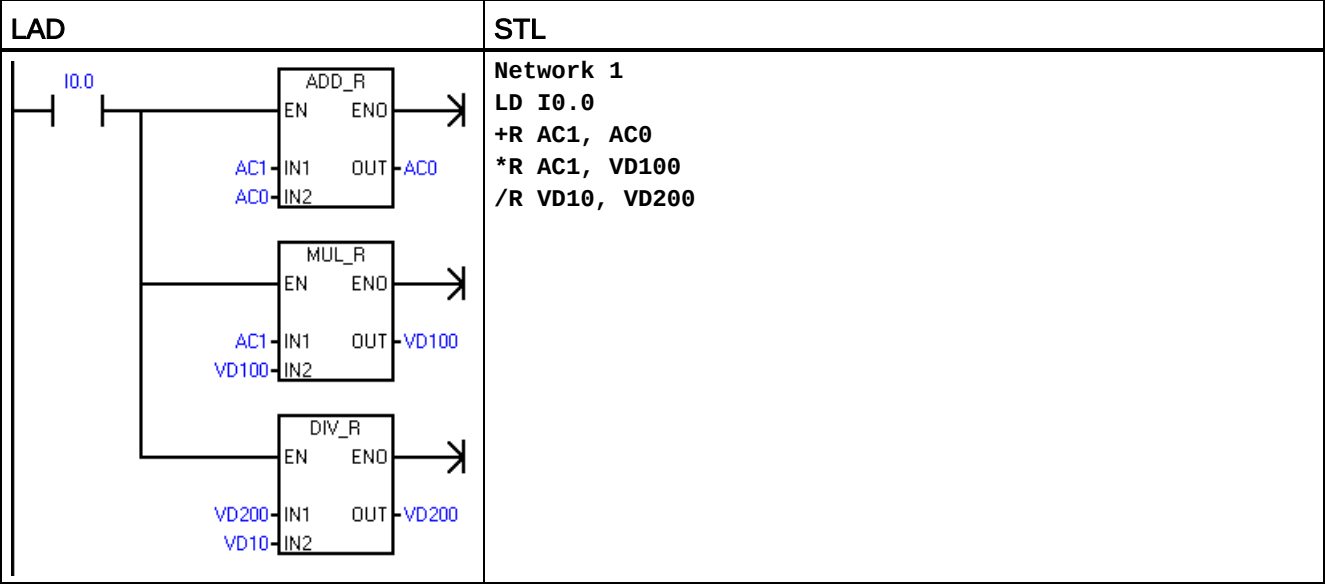
LAD 示例中的实数运算
