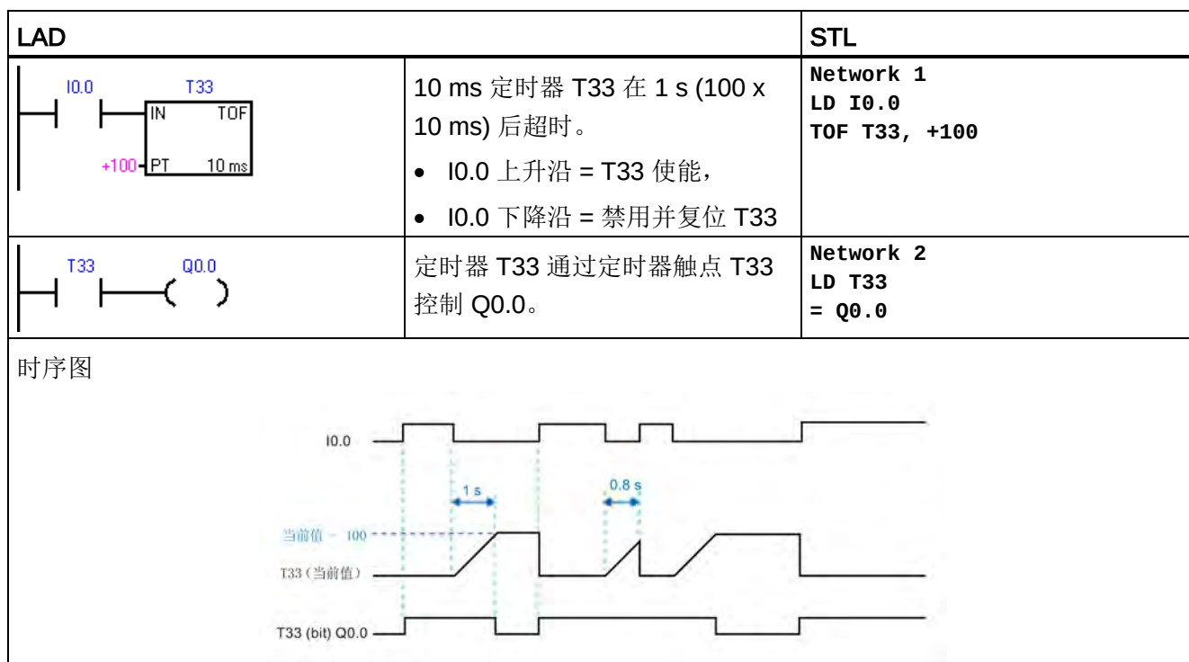
TOF 断开延时定时器示例
