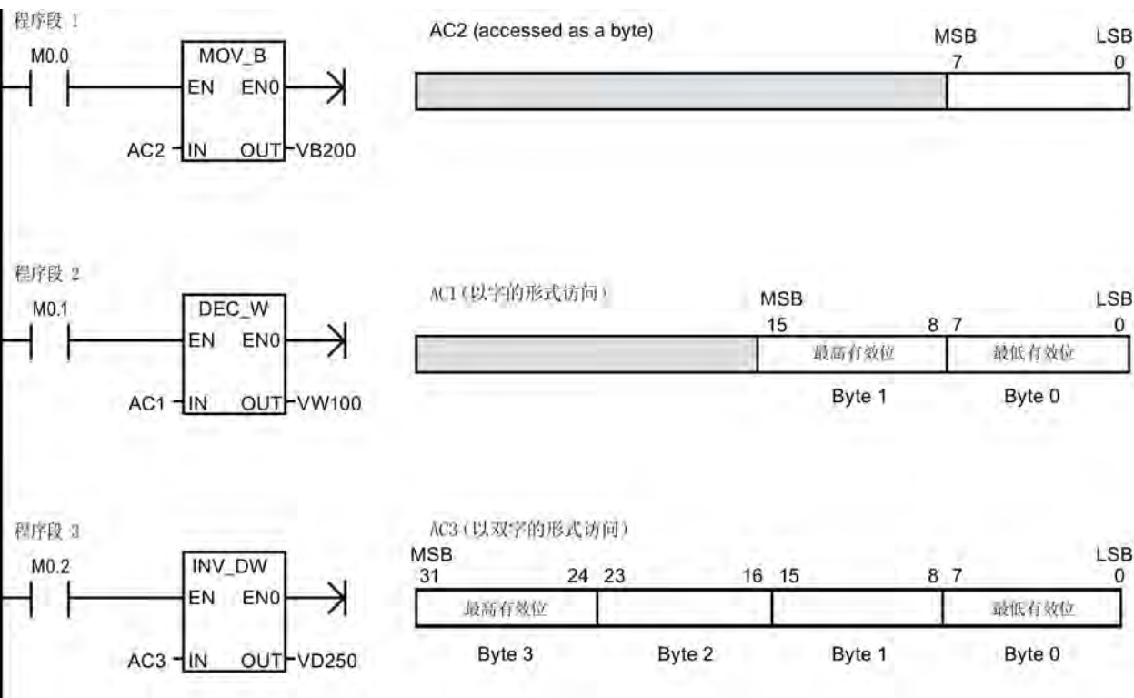
图 4-4 访问累加器
