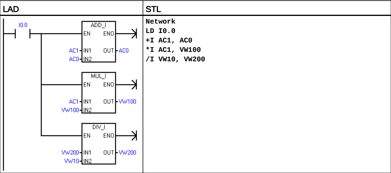
LAD 示例中的整数运算
