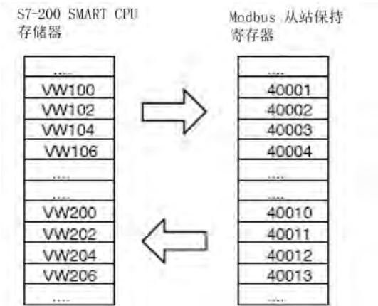
图 9-1 程序数据传送示例
