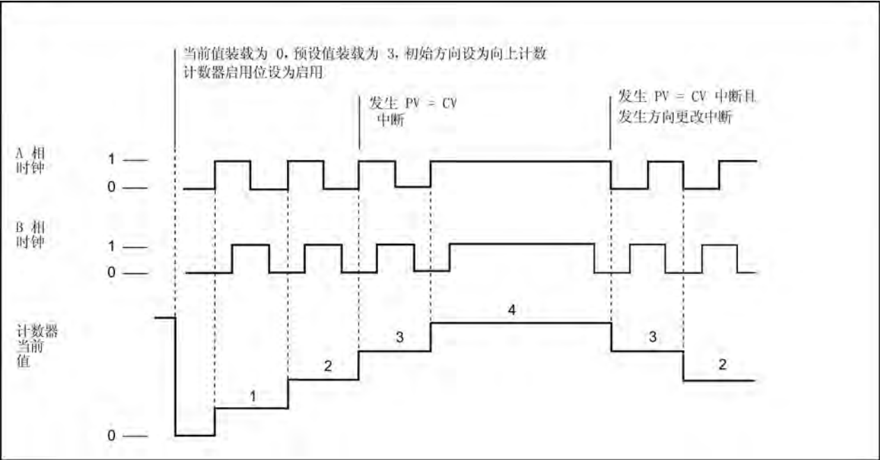
HSC 模式 9 和 10 (AB 正交相 1x)
