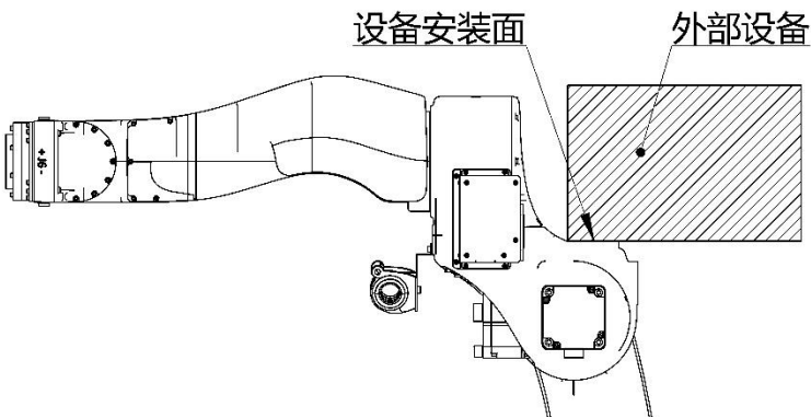
图 9-6 AIR6-1450A 操作机肘部负载安装尺寸示意图
