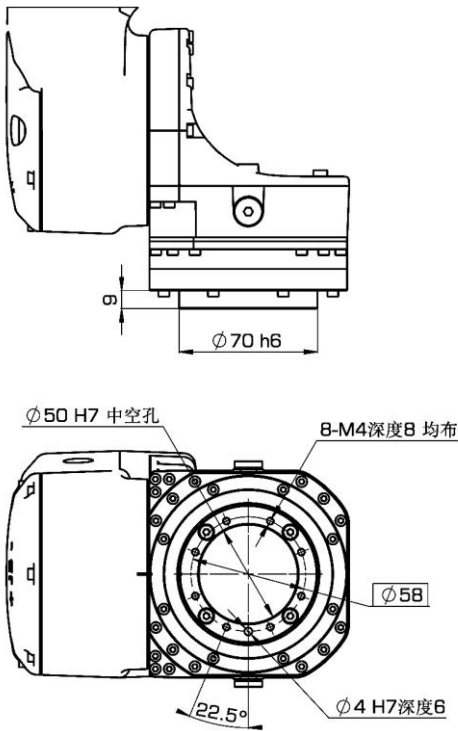
图 9-3 AIR6-1450A 操作机腕部法兰尺寸示意图
