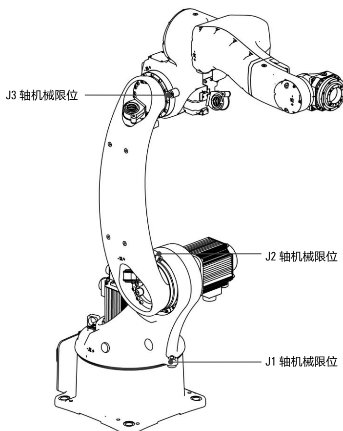
图 9-2 AIR6-1450A 操作机上机械式制动器
