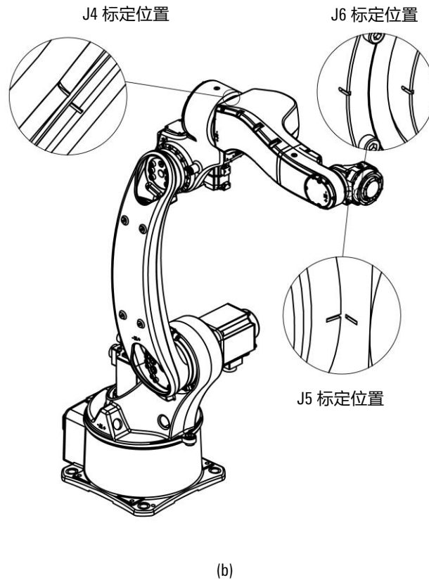
图 10-1 AIR6-1450A 各轴零点示意图
