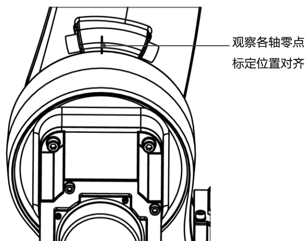
图 10-2 肉眼观察零点标定方式
