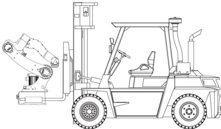
图 4-4 AIR6-1450A 叉车搬运示意图
