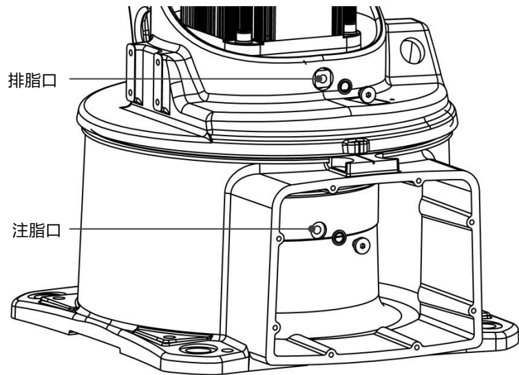
图 13-8 更换 J1 轴减速器润滑脂
