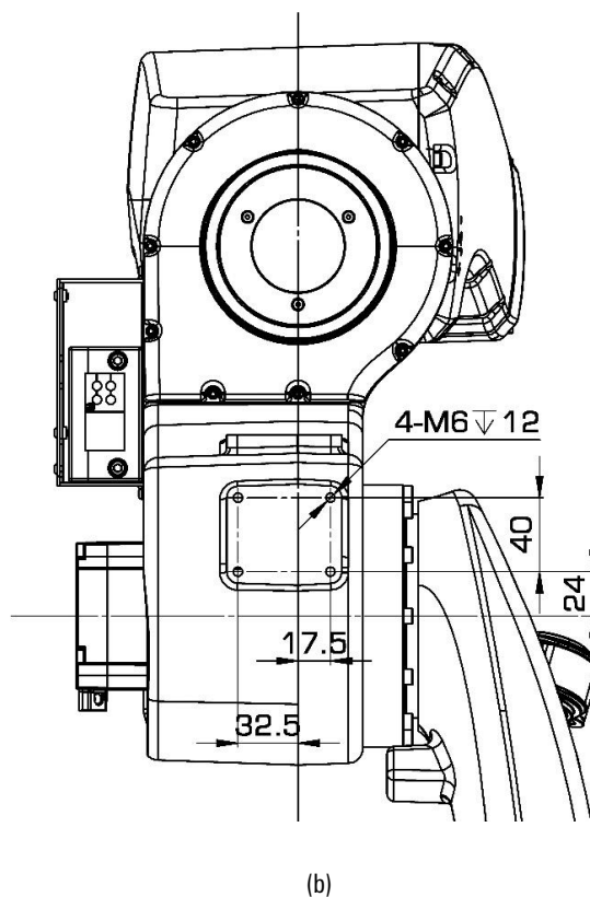
图 9-7 AIR6-1450A 操作机肘部负载接口尺寸示意图
