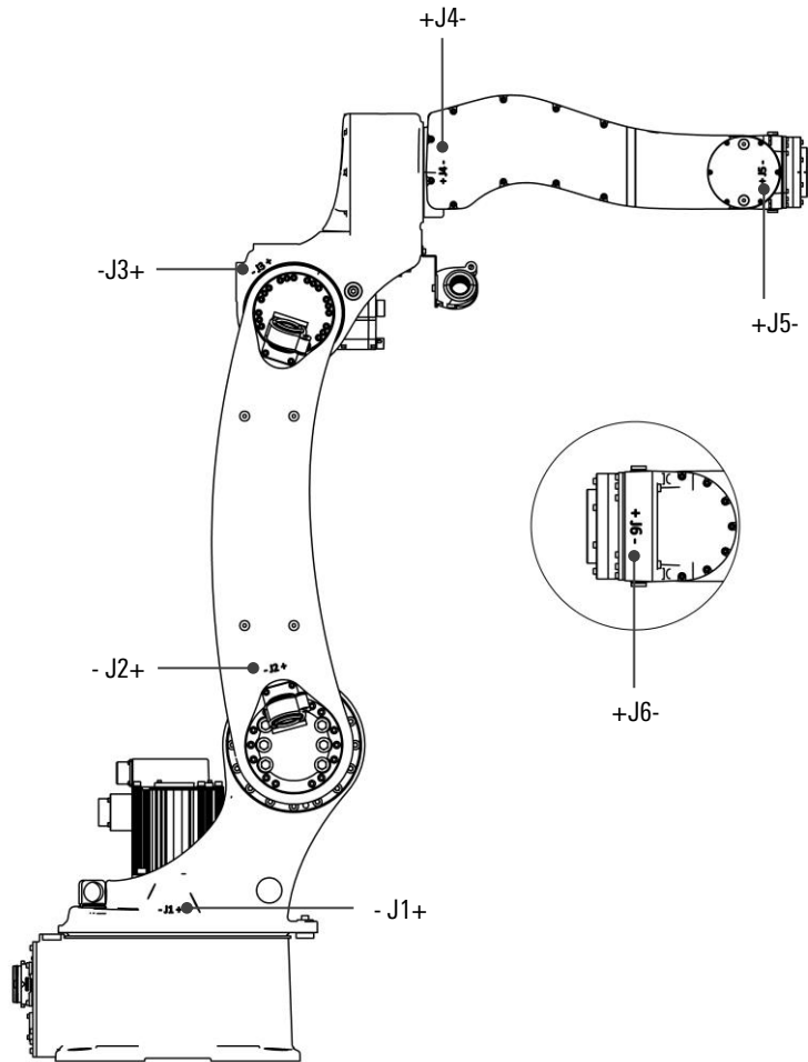
图 3-5 AIR6-1450A 操作机上各轴方向标识
