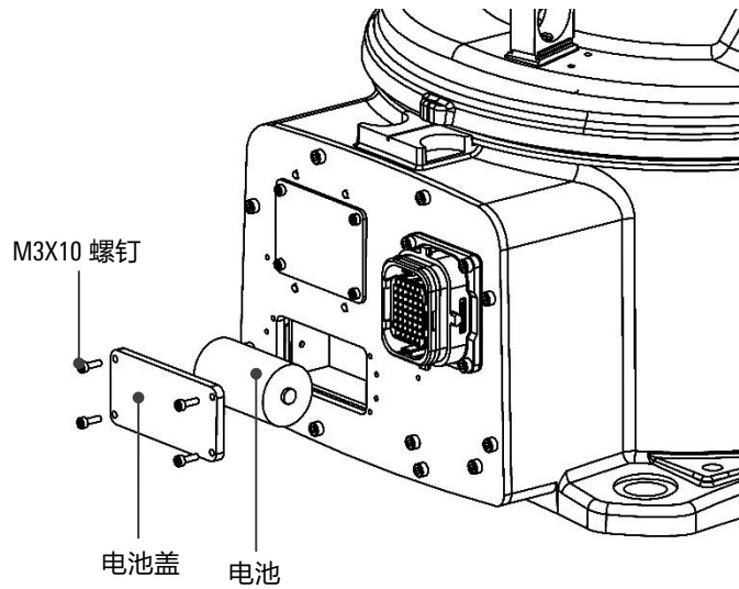
图 13-4 更换电池
