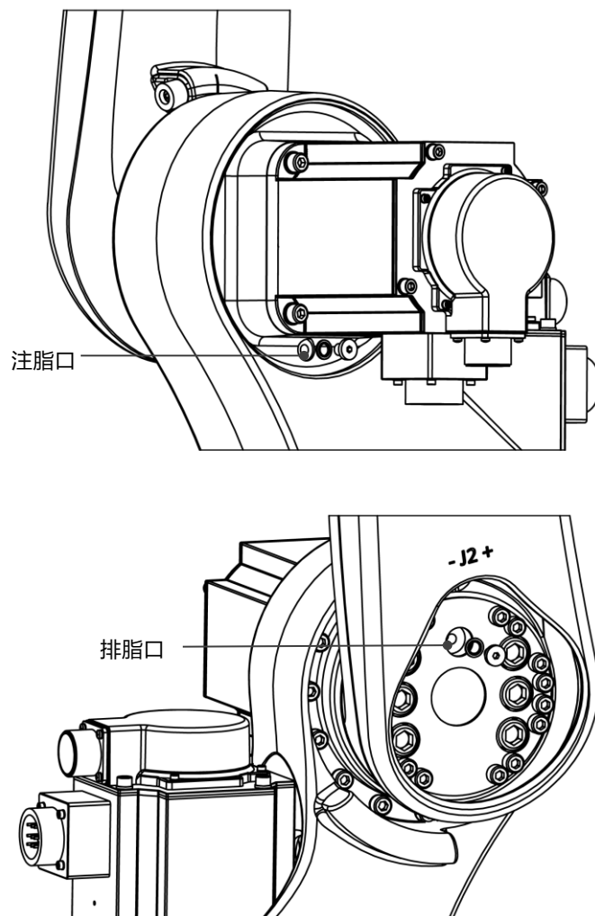
图 13-9 更换 J1 轴减速器润滑脂
