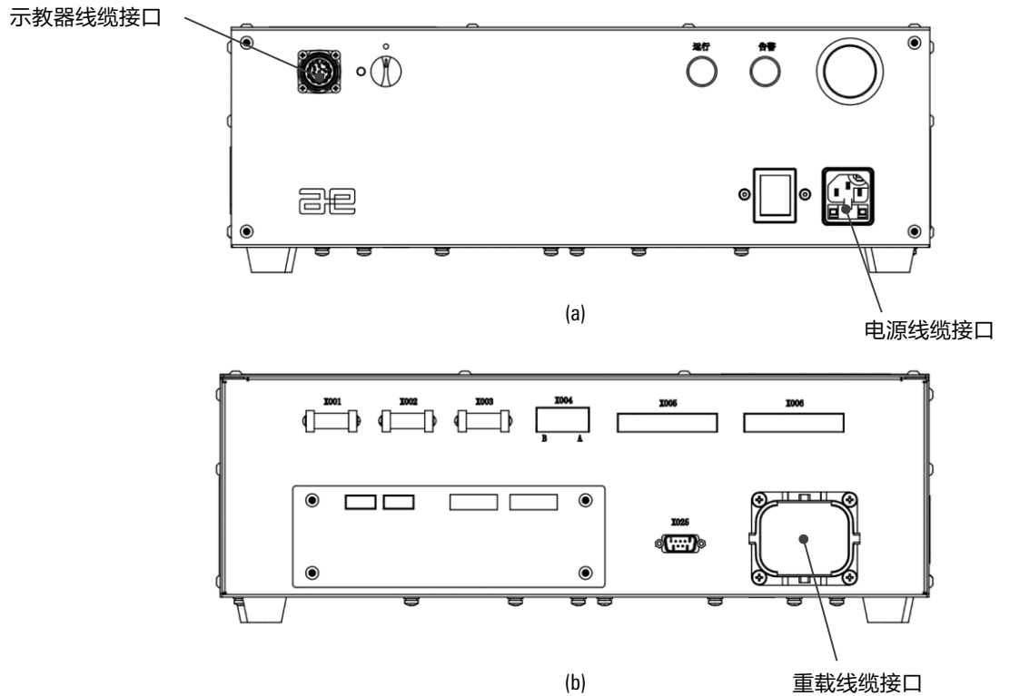
图 8-4 AIR6-1450A 控制柜线缆连接器定义
