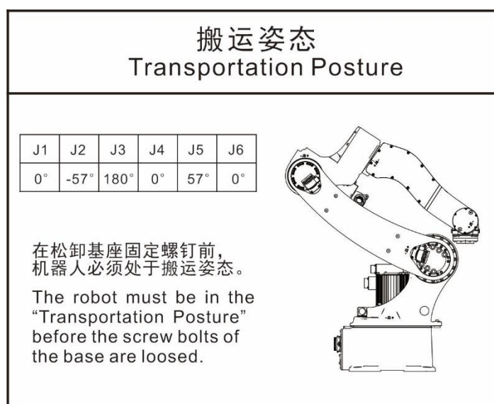
图 3-4 AIR6-1450A 本体各轴搬运姿态标签
