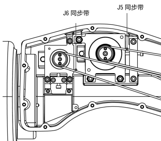
图 13-7 更换 J5/J6 轴同步带示意图
