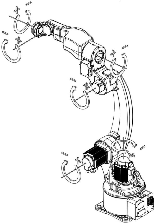
图 10-3 操作机各轴的运动方向
