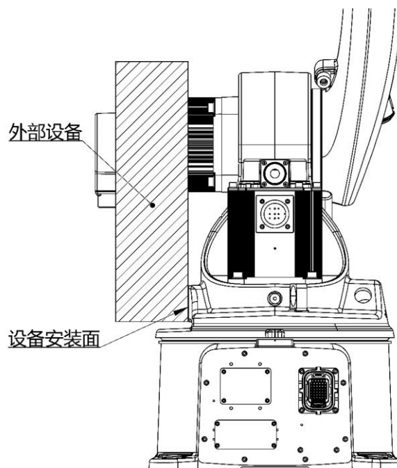
图 9-8 AIR6-1450A 操作机肩部负载安装尺寸示意图
