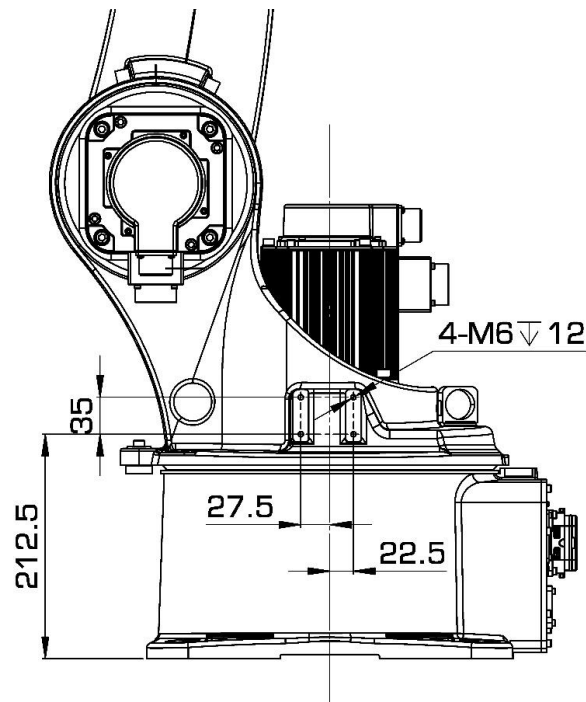
图 9-9 AIR6-1450A 操作机肘部负载接口尺寸示意图
