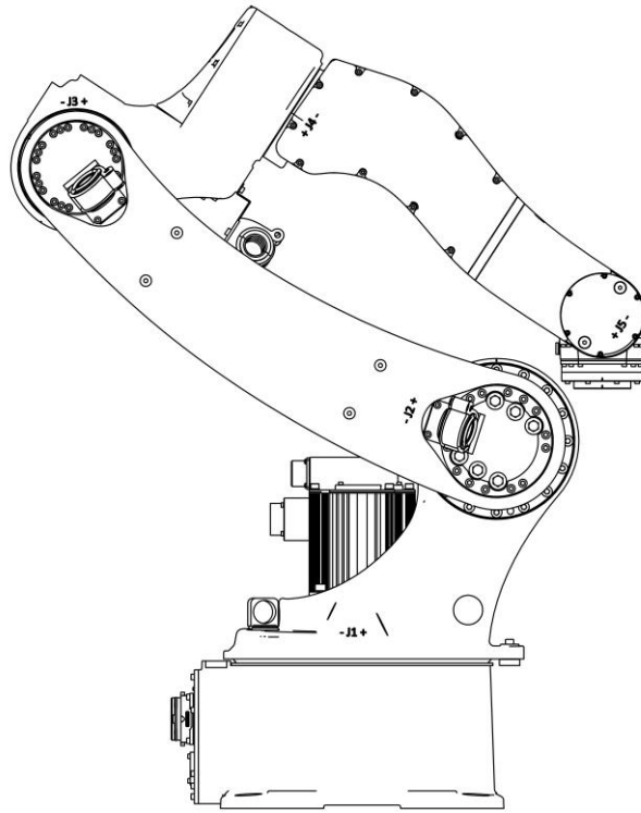
图 4-2 AIR6-1450A 操作机搬运位姿图
