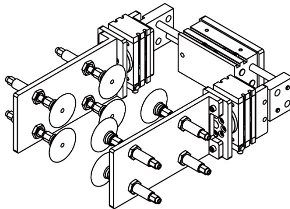
图 8-2 工业机器人用吸盘
