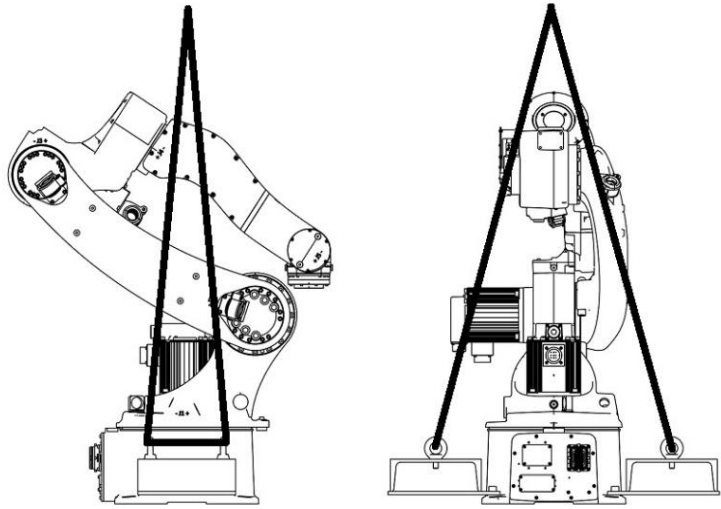
图 4-5 AIR6-1450A 吊环搬运示意图
