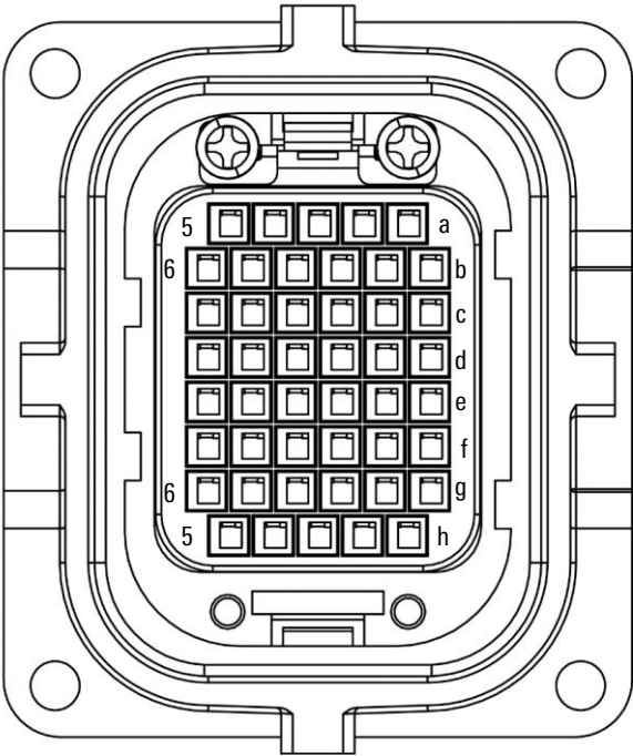
图 7-2 AIR6-1450A 型操作机重载接口示意图
