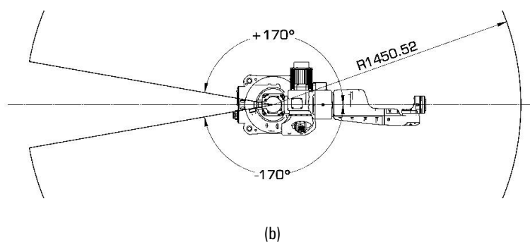
图 9-1 AIR6-1450A 操作机工作范围
