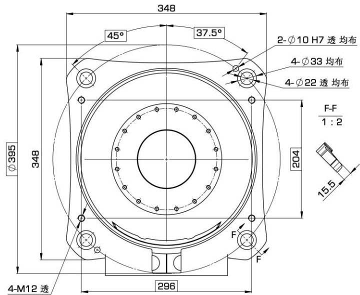
图 6-1 AIR6-1450A 操作机基座接口尺寸
