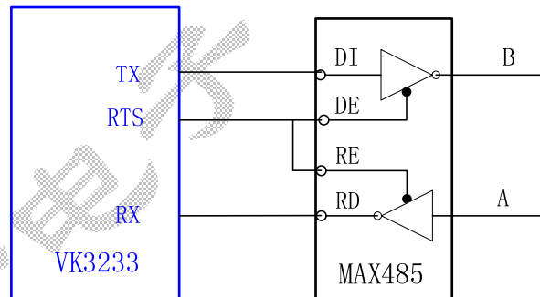
图 11.5.1 RS485 连接图
