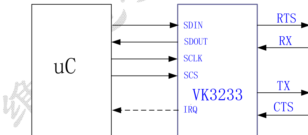
图 9.1 SPI 与主机连接图
