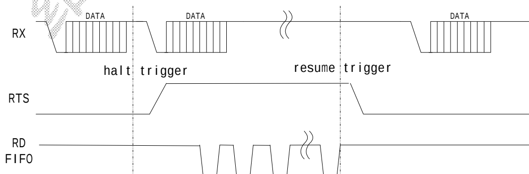
图 11.3.2.2 硬件流量操作时序图
