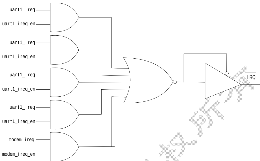
图 8.3 VK3233 中断结构图
