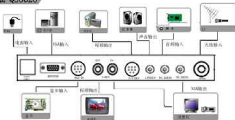
产品连接图 QS8628
