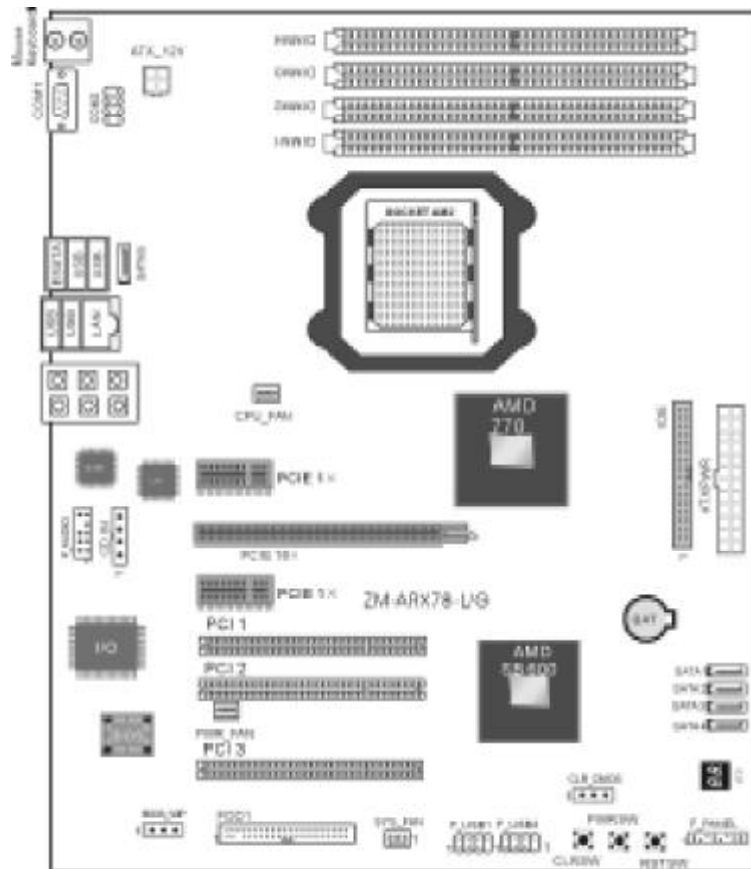
ZM-ARX78-L/G 主机板布局图
