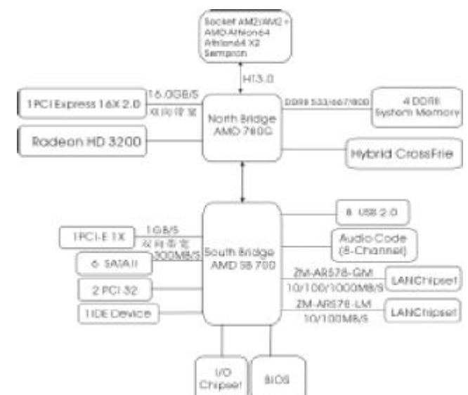
AMD 780G+SB700 芯片组图
