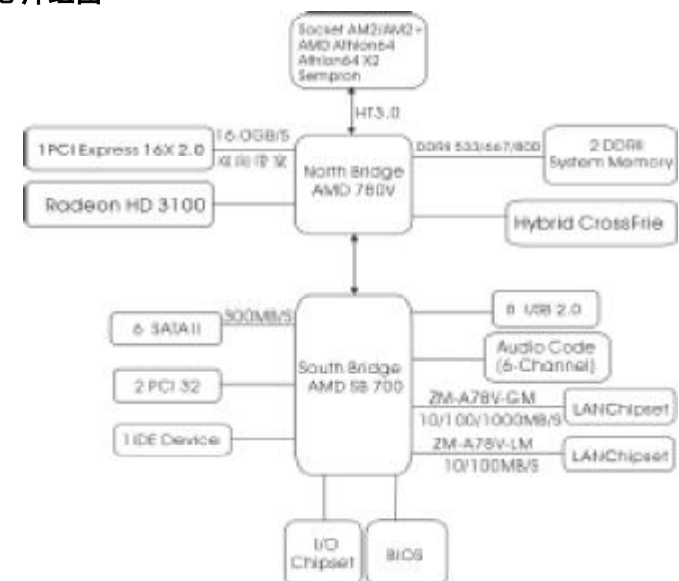
AMD 780V+SB700 芯片组图
