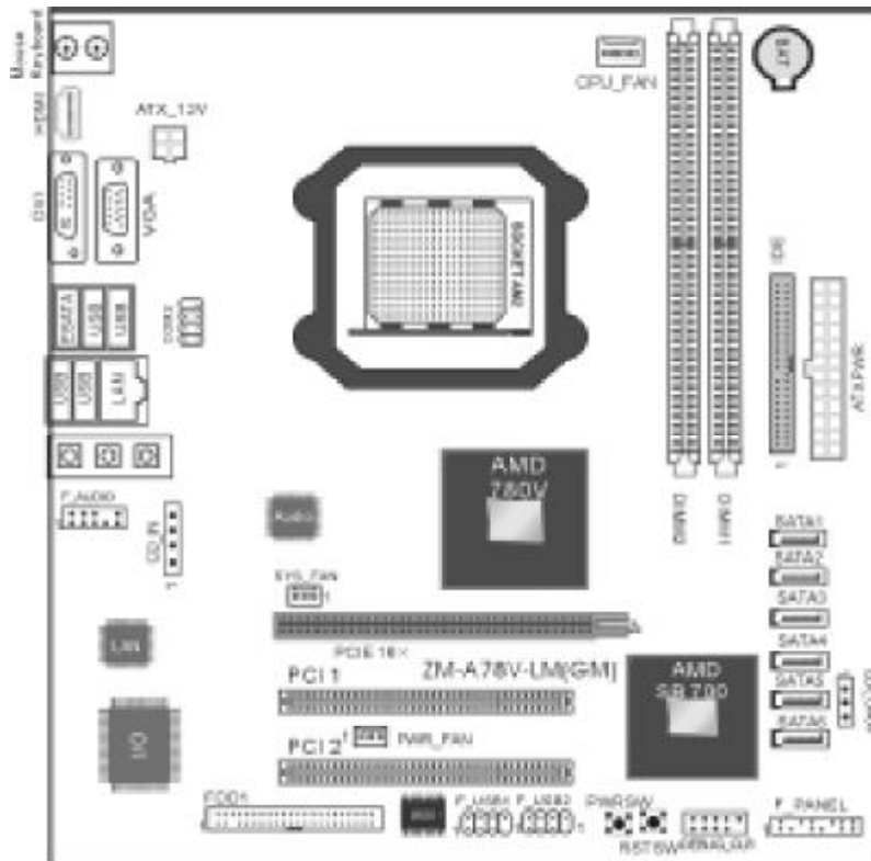
ZM-A78V-LM (GM) 主机板布局图
