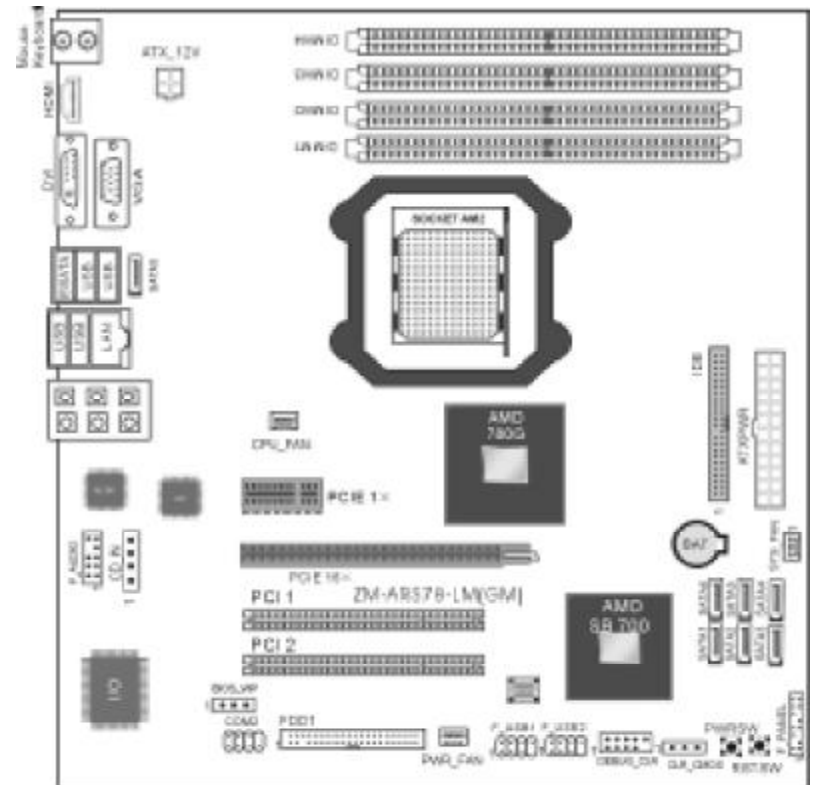
ZM-ARS78-LM (GM) 主机板布局图
