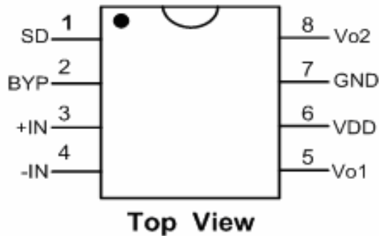
XPT8002 的各种封装管脚
