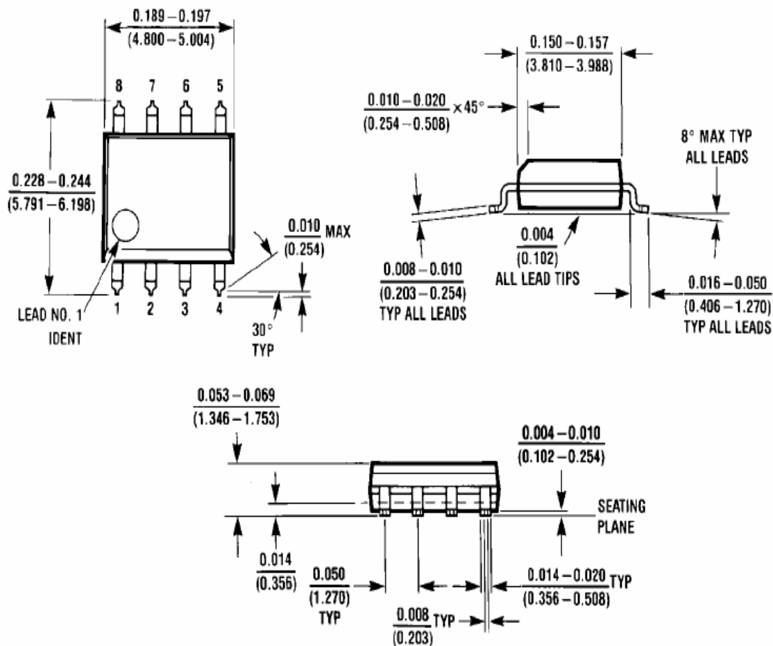
图3 SOP封装尺寸图
