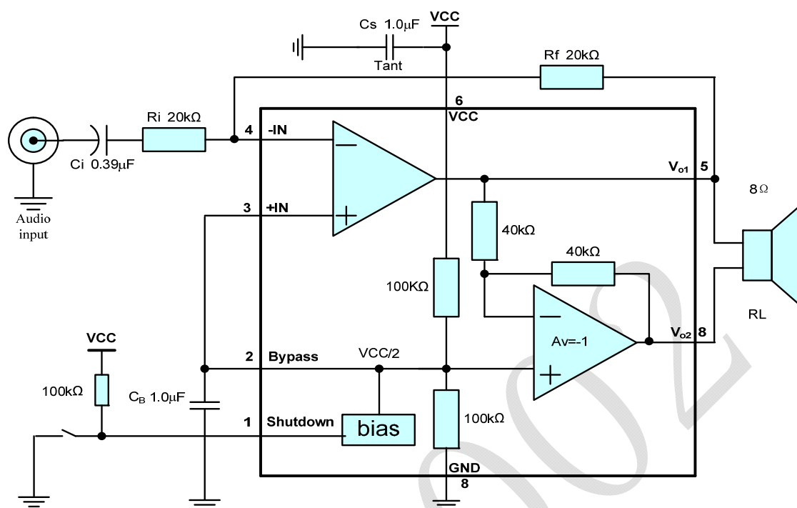
XPT8002 典型应用电路
