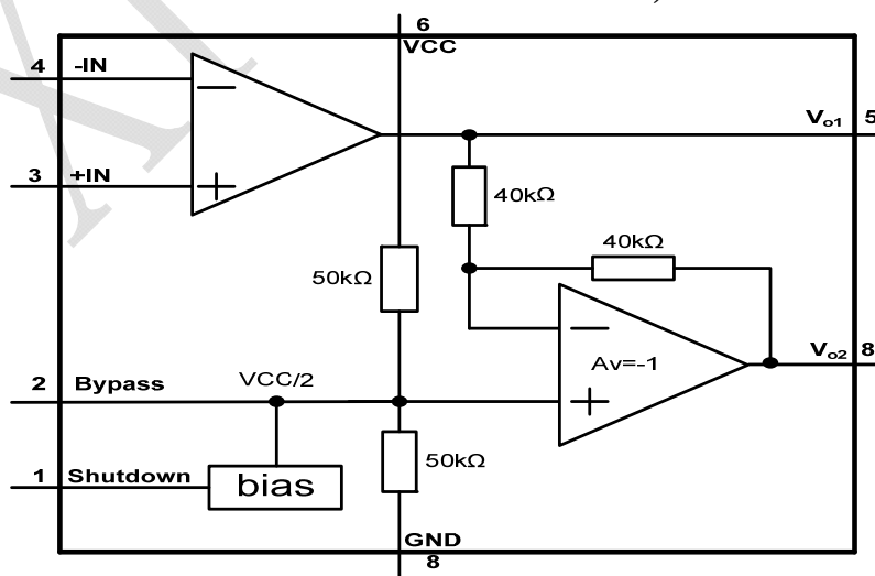
图1 XPT8002 原理框图
